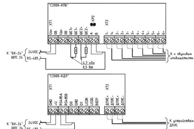
Типовая схема подключения адресных устройств в линию RS-485
