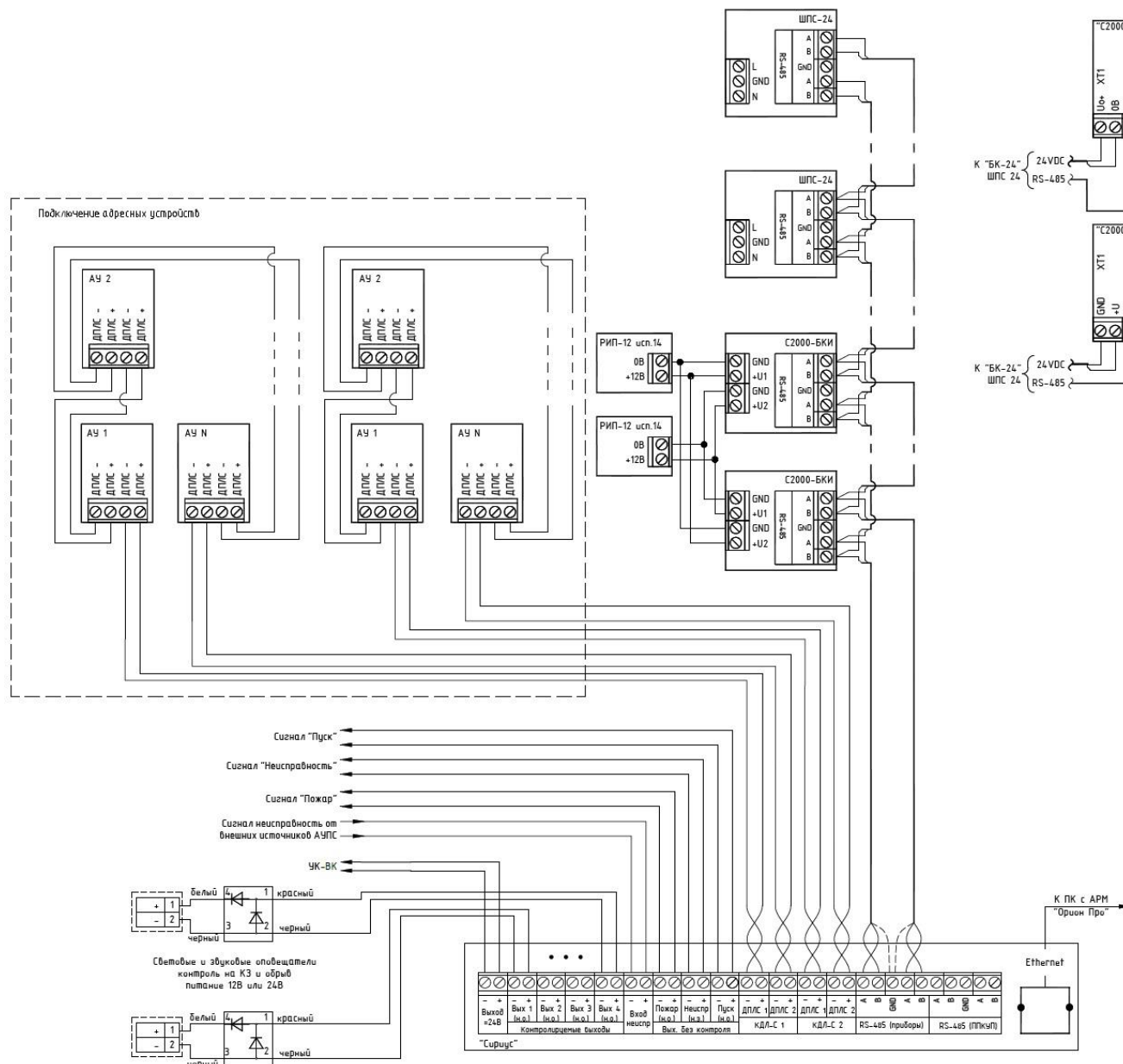
Типовая схема подключения адресных устройств ДПЛС, RS-485 к прибору приема контроля и управления охранно-пожарному ППКУОП "Сирius"
