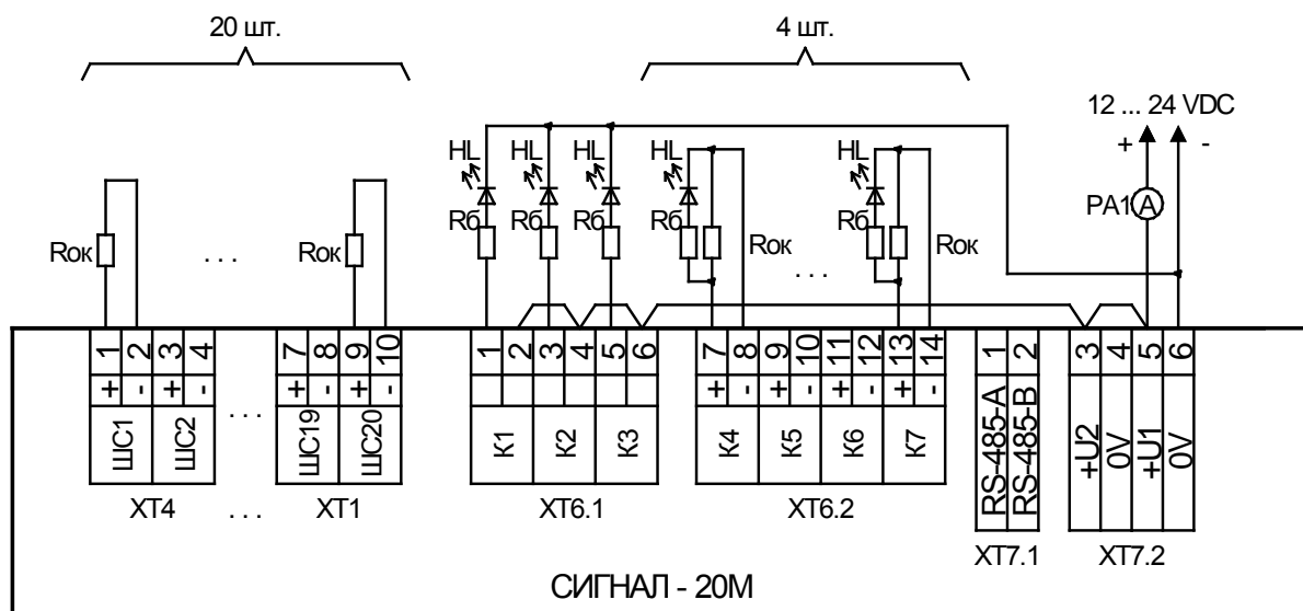
Рисунок 3.4.1. Схема подключения при полной проверке,
