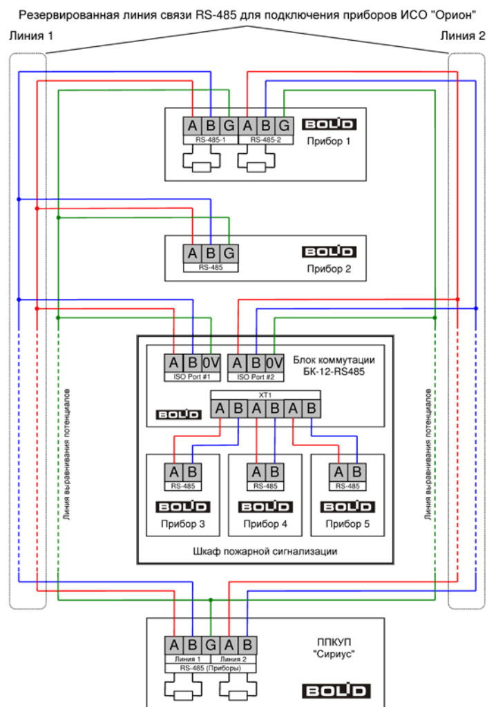
Рисунок 59. Схема подключения дополнительных блоков и приборов ИСО «Орион»
