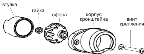
Рисунок 3 – Конструкция кронштейна
