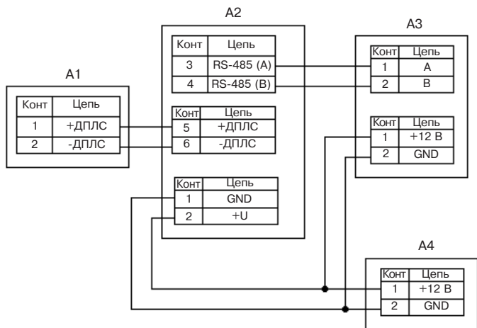
Рисунок 4 – Клеммы подключения
