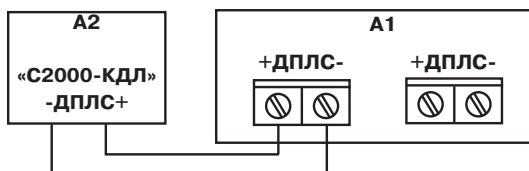
Рисунок 7 – Клеммы подключения
