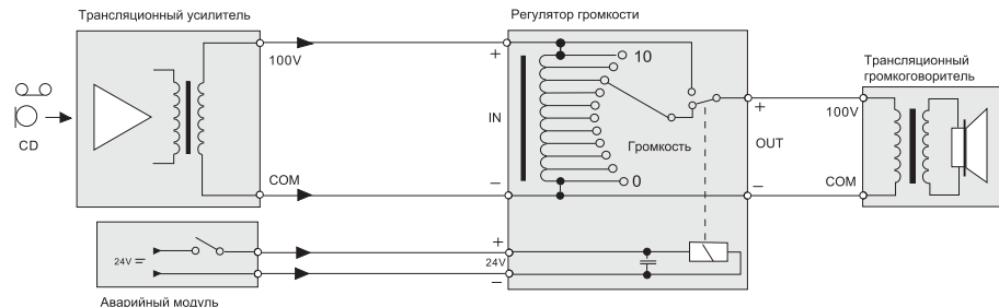
Схема подключения
