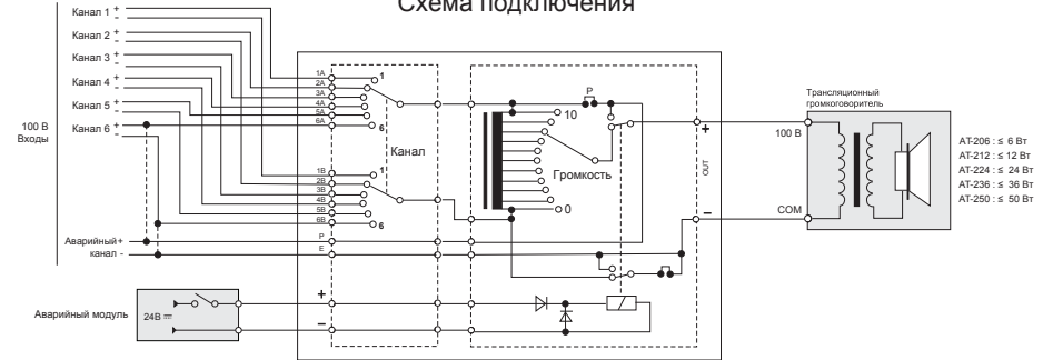
Схема подключения
