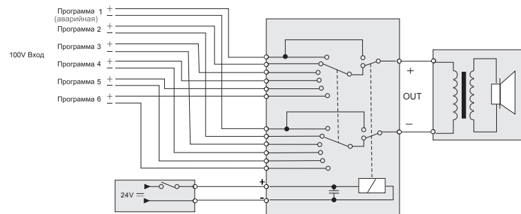
Схема подключения
