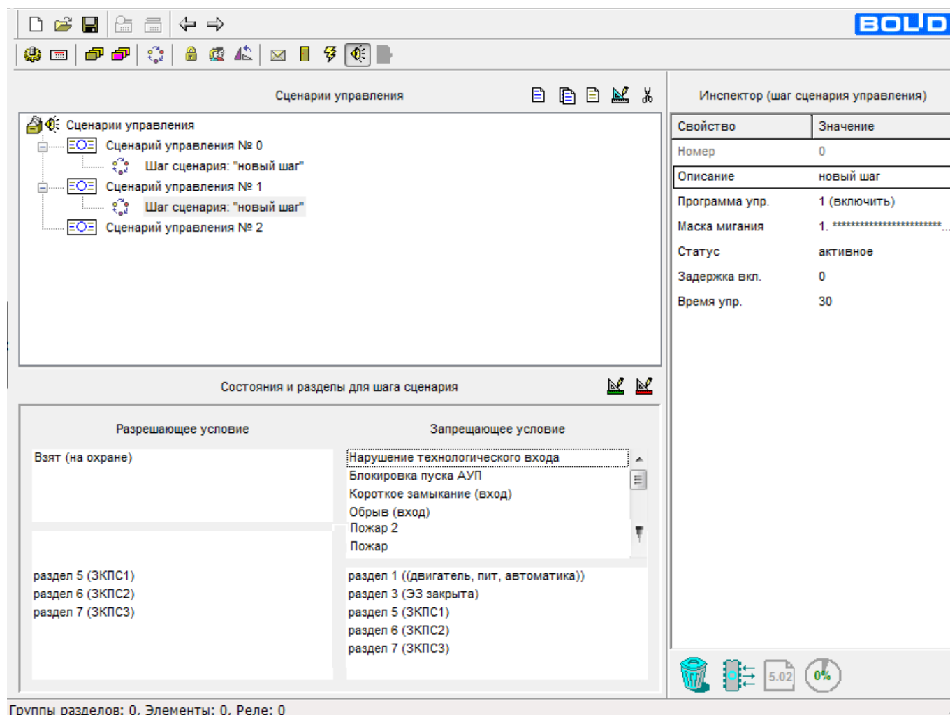
Рисунок 14. Настройка сценария управления реле 4
