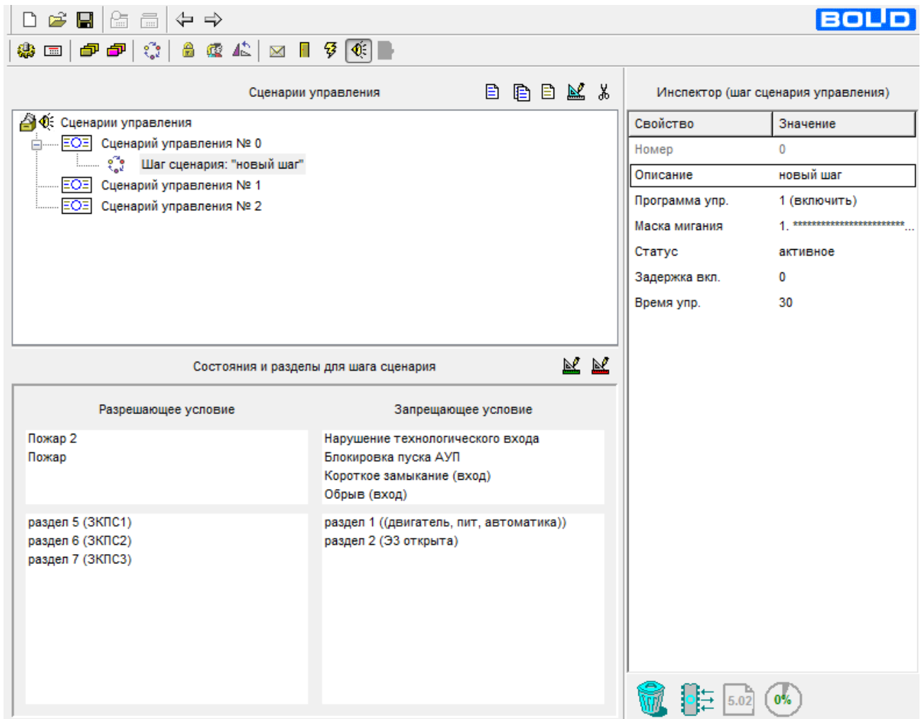
Рисунок 12. Настройка сценария управления реле 3
