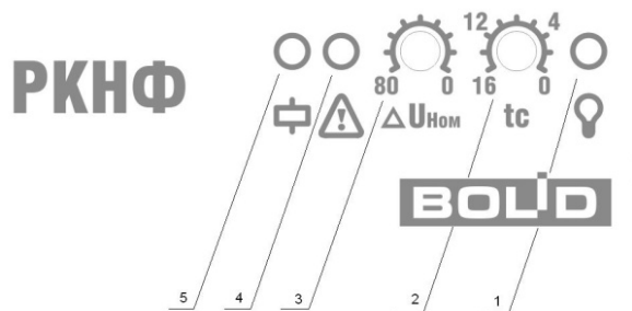
Рисунок 24. Лицевая панель РКНФ
