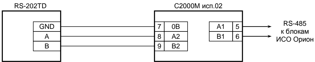
RS-202TD – радиопередатчик «Риф Стринг RS-202TD-RR»; C2000M исп.02 - пульт контроля и управления «C2000M исп.02».
