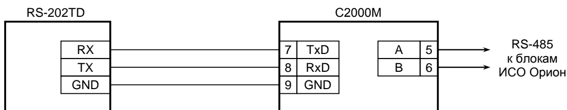
RS-202TD – радиопередатчик «Риф Стринг RS-202TD-RR»; C2000M - пульт контроля и управления «С2000М».
