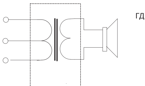
СОГЛАСУЮЩИЙ ТРАНСФОРМАТОР
