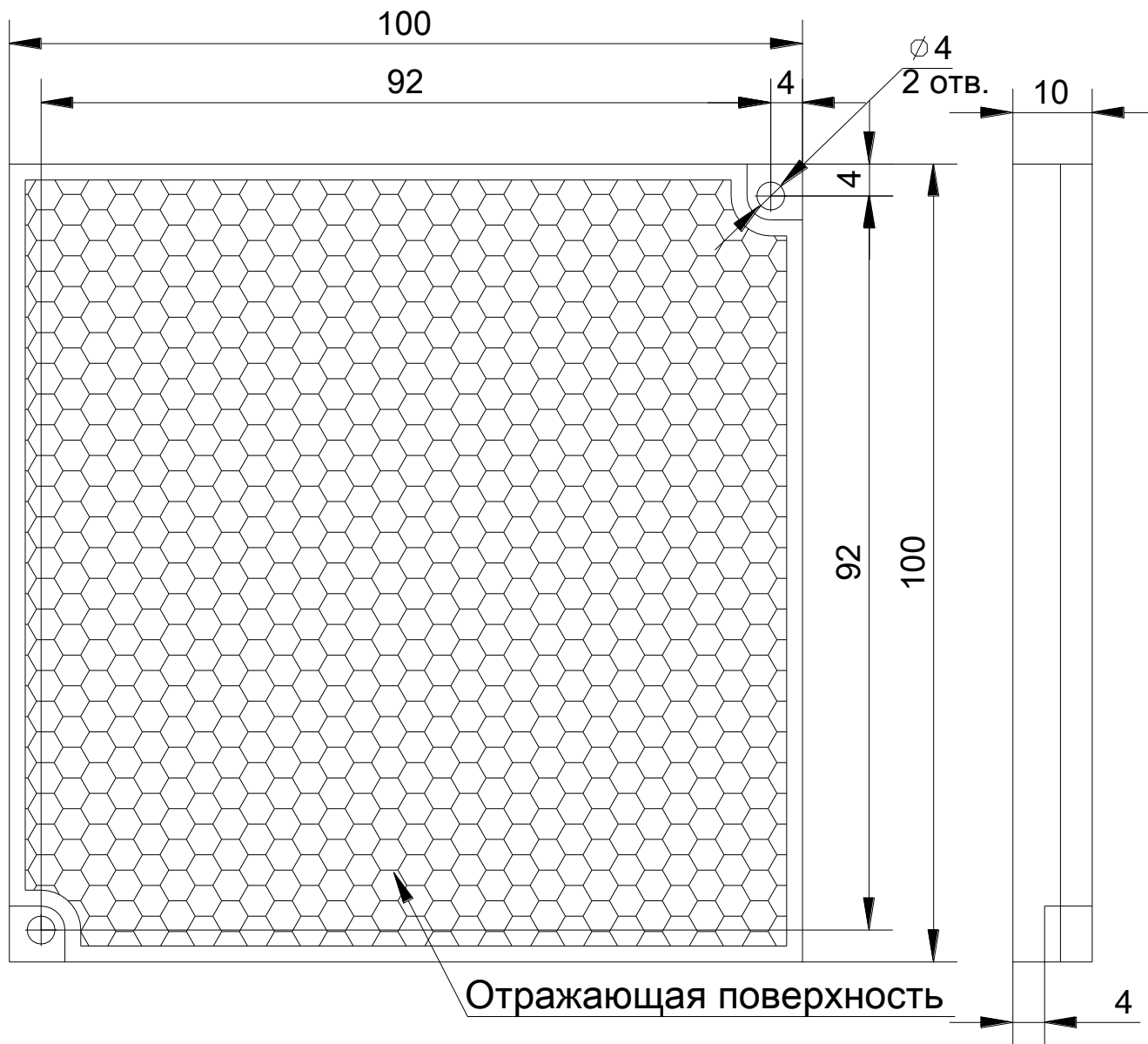
Рисунок 1 Общий вид отражателя
