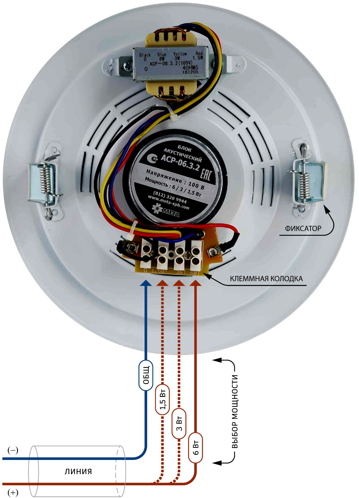
Рис.. 3 Схема подключения БА
