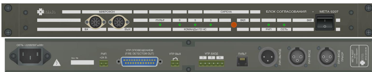
Рисунок 1. Внешний вид БС (лицевая и задняя панель).
