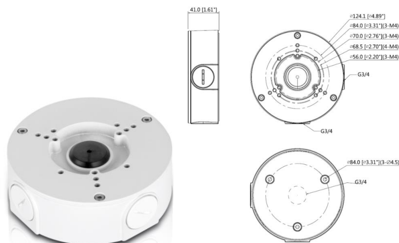
Рисунок 5.3 — Монтажная коробка BR-204
