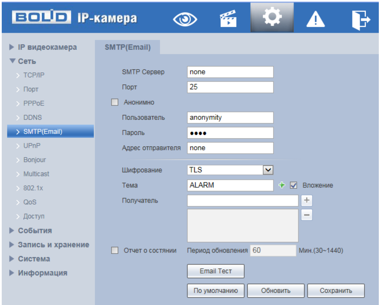
Рисунок 7.57 — Подпункт меню «SMTP»
