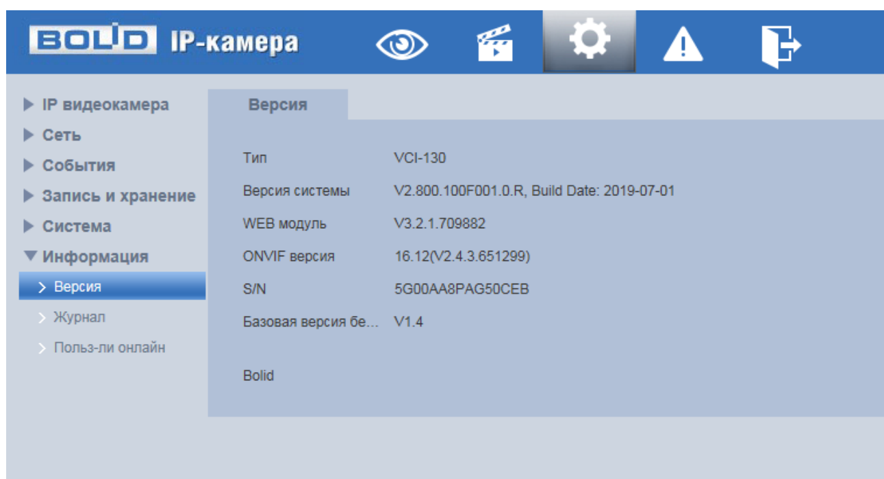
Рисунок 7.121 — Подпункт меню «Версия»
