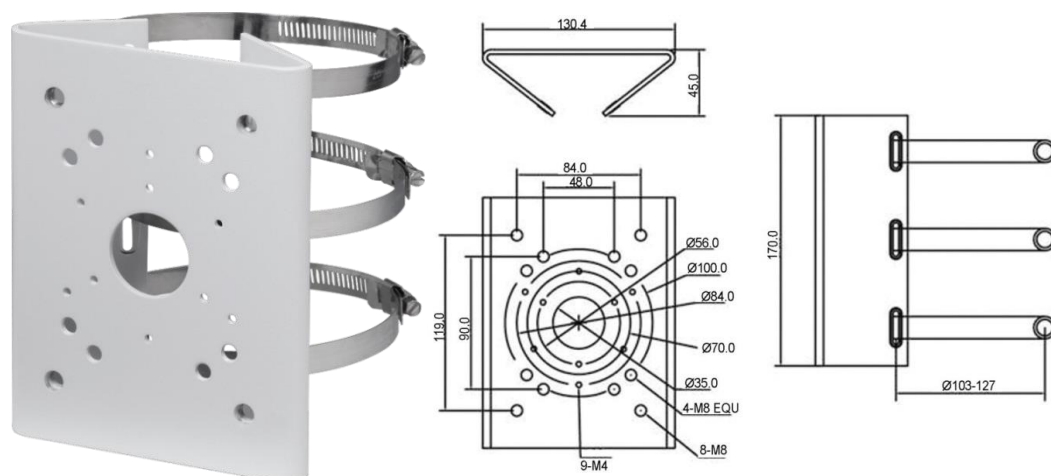
Рисунок 5.11 — Столбовой кронштейн BR-103
