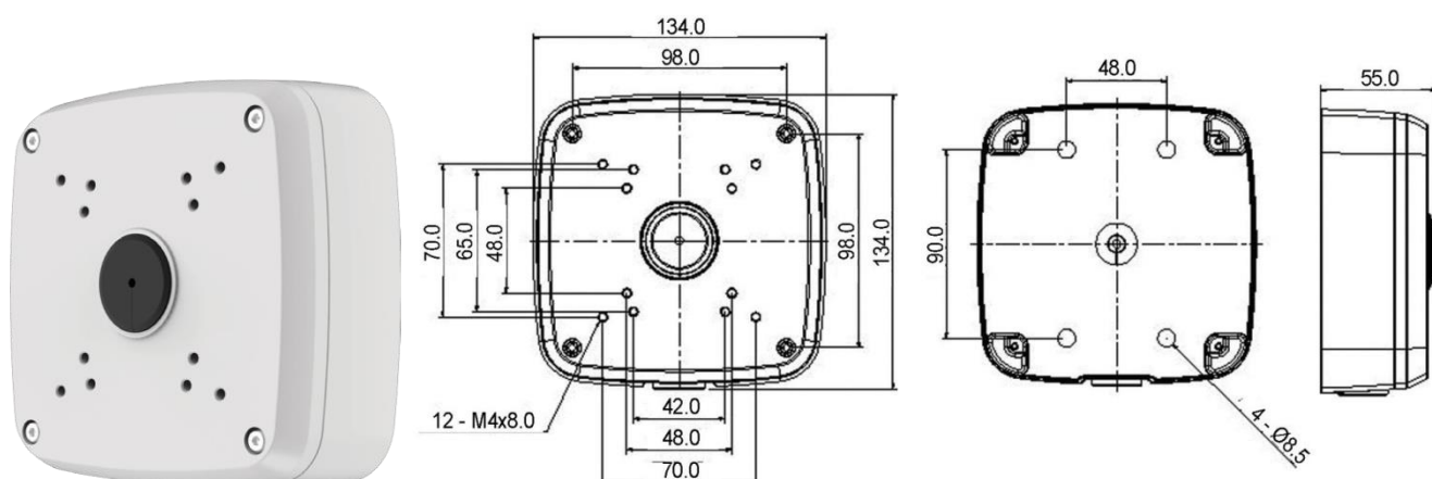
Рисунок 5.3 — Монтажная коробка BR-201
