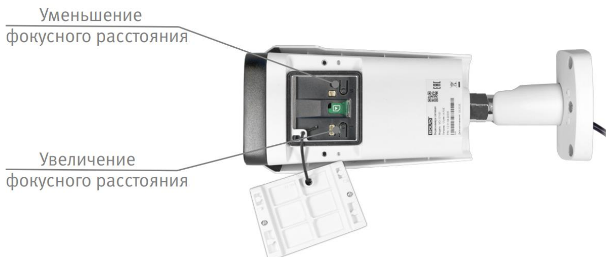
Рисунок 5.14 — Настройка фокусного расстояния вручную
