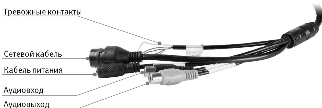
Рисунок 6.1 — Кабель видеочамеры
