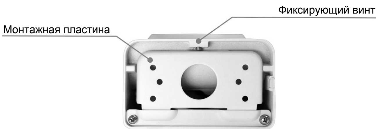
Рисунок 5.5 — Настенный кронштейн
