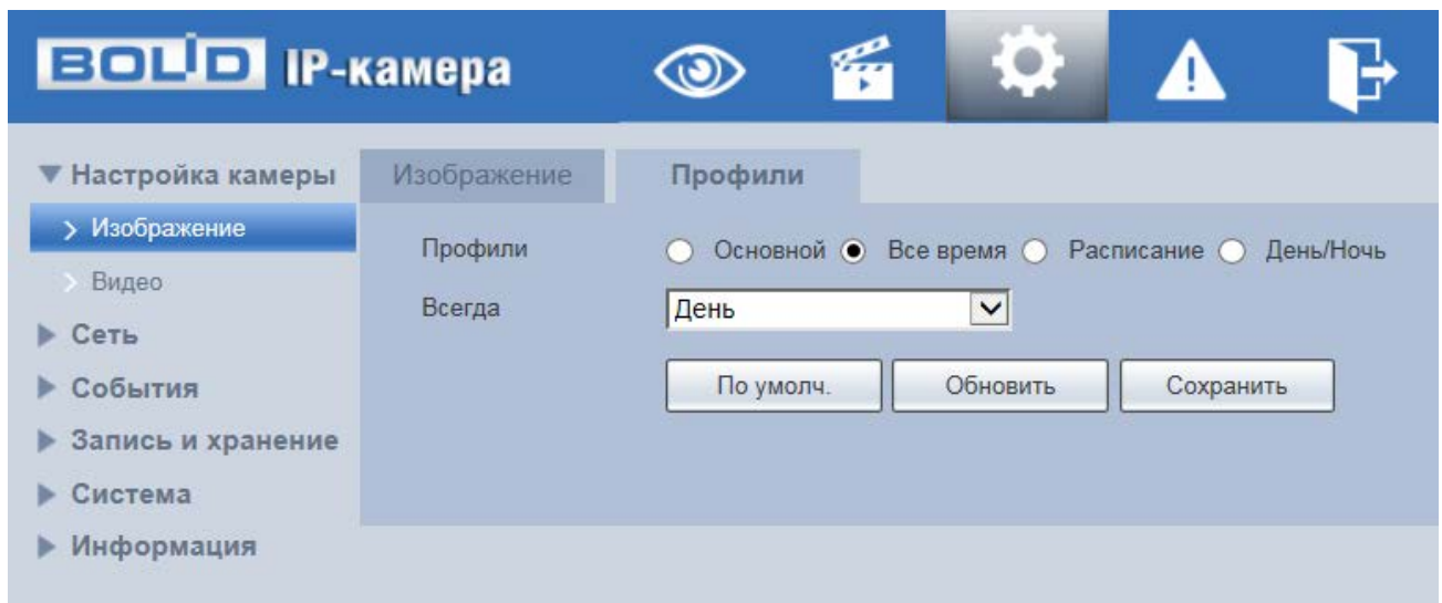
Рисунок 7.36 — Вкладка «Профили»
