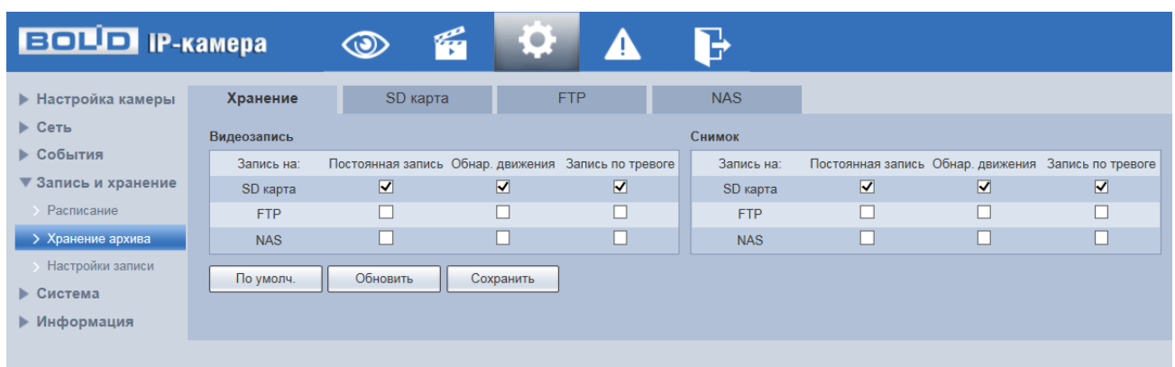
Рисунок 7.101 — Вкладка «Хранение»
