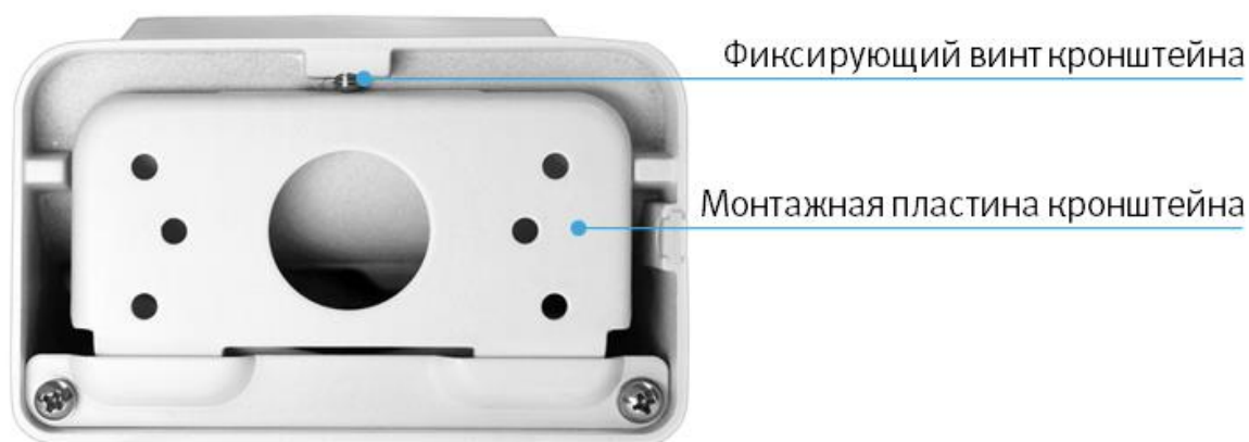
Рисунок 5.8 – Настенный кронштейн
