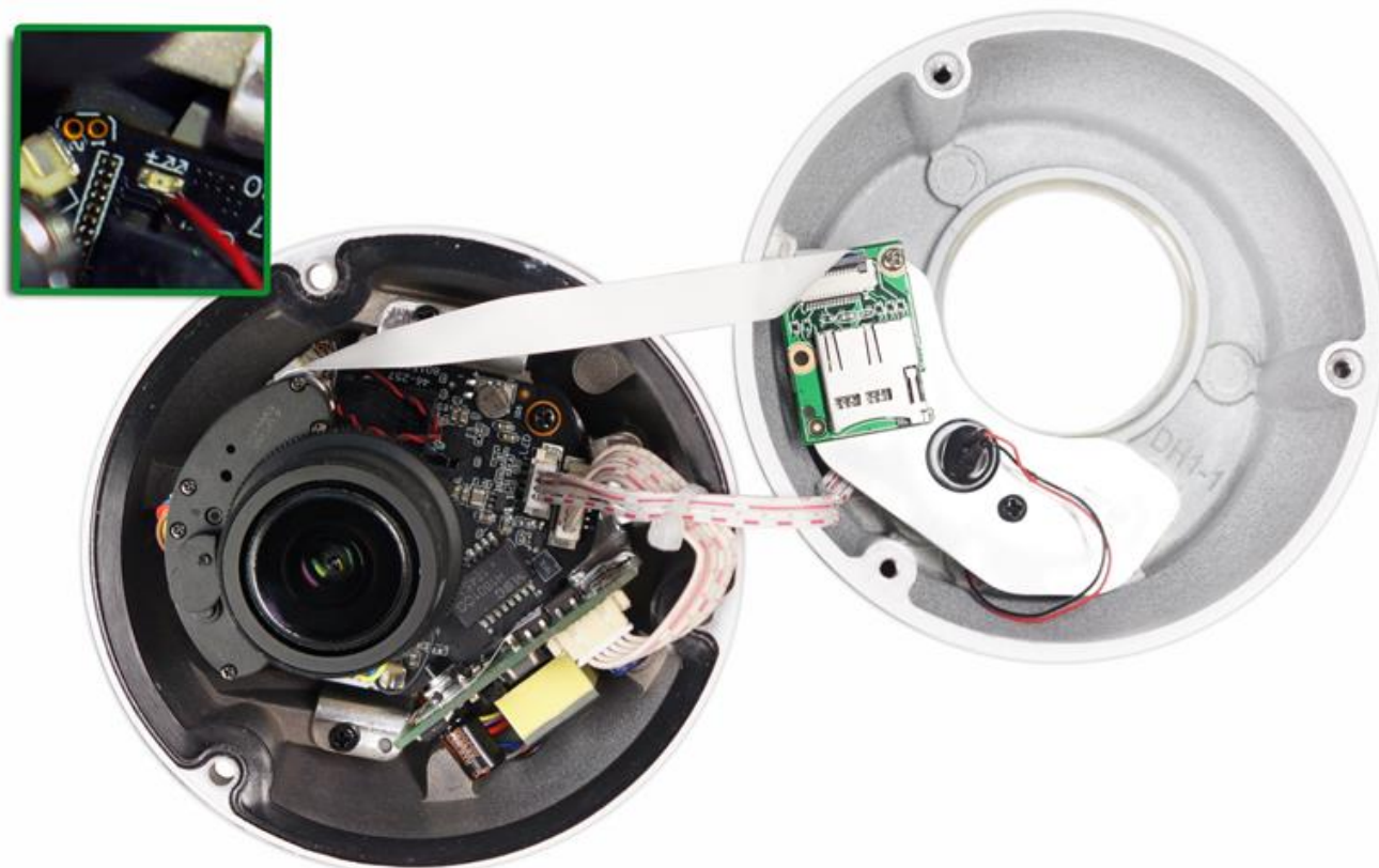
Рисунок 4.2 – Расположение кнопки аппаратного сброса и слота для карты памяти
