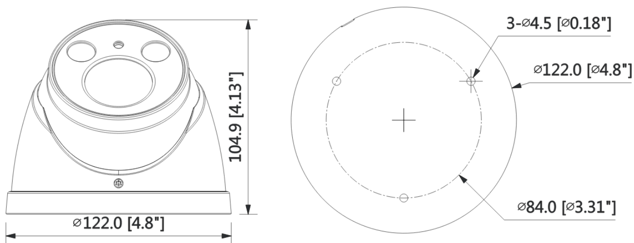
Рисунок 5.1 – Габаритные размеры видеокамеры
