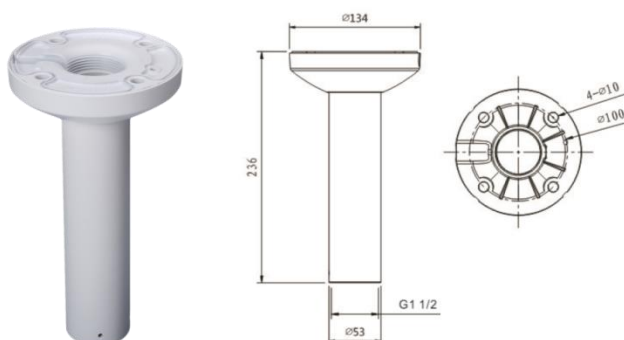
Рисунок 5.2 – Потолочный кронштейн BR-104
