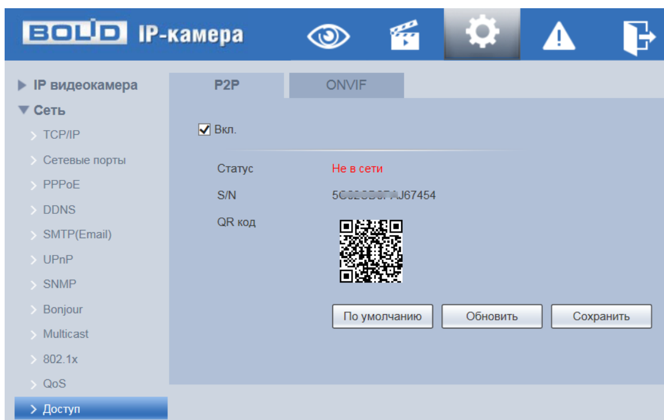
Рисунок 7.74 — Вкладка «P2P»
