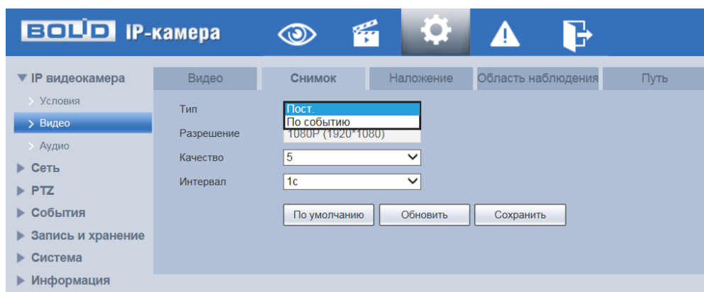
Рисунок 7.43 — Вкладка «Снимок»
