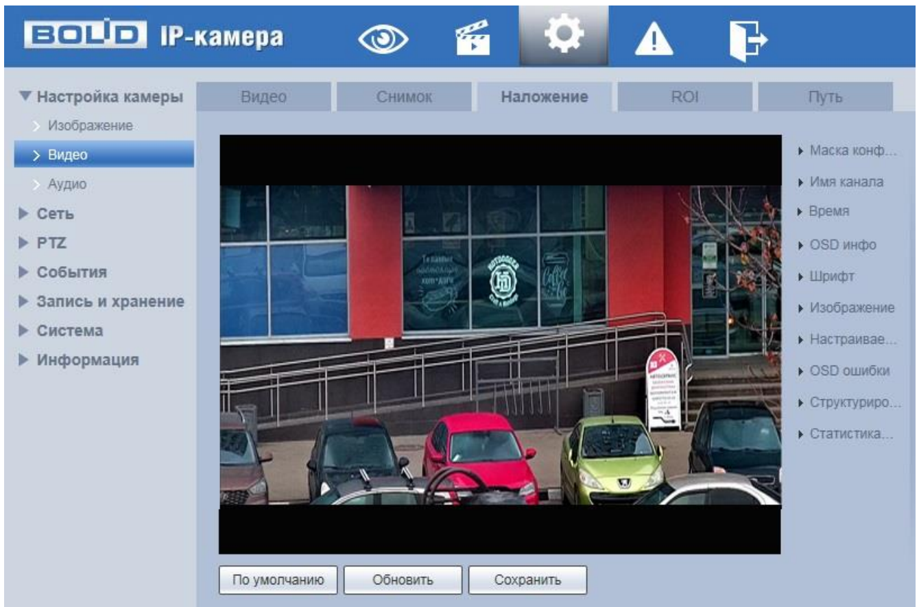
Рисунок 7.44 — Вкладка «Наложение»
