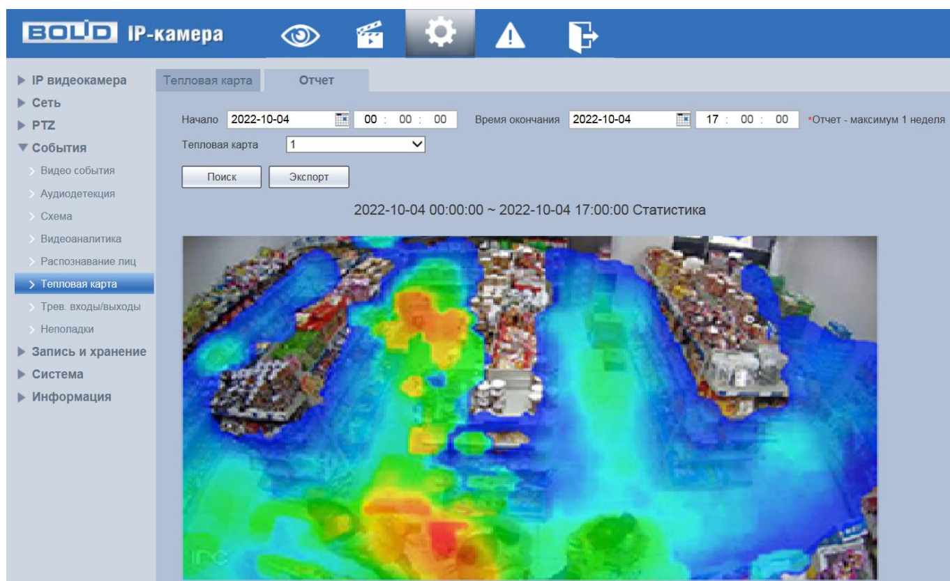
Рисунок 7.115 – Вкладка «Отчет»
