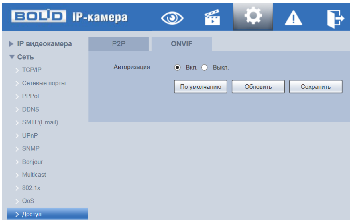
Рисунок 7.75 — Вкладка «ONVIF»
