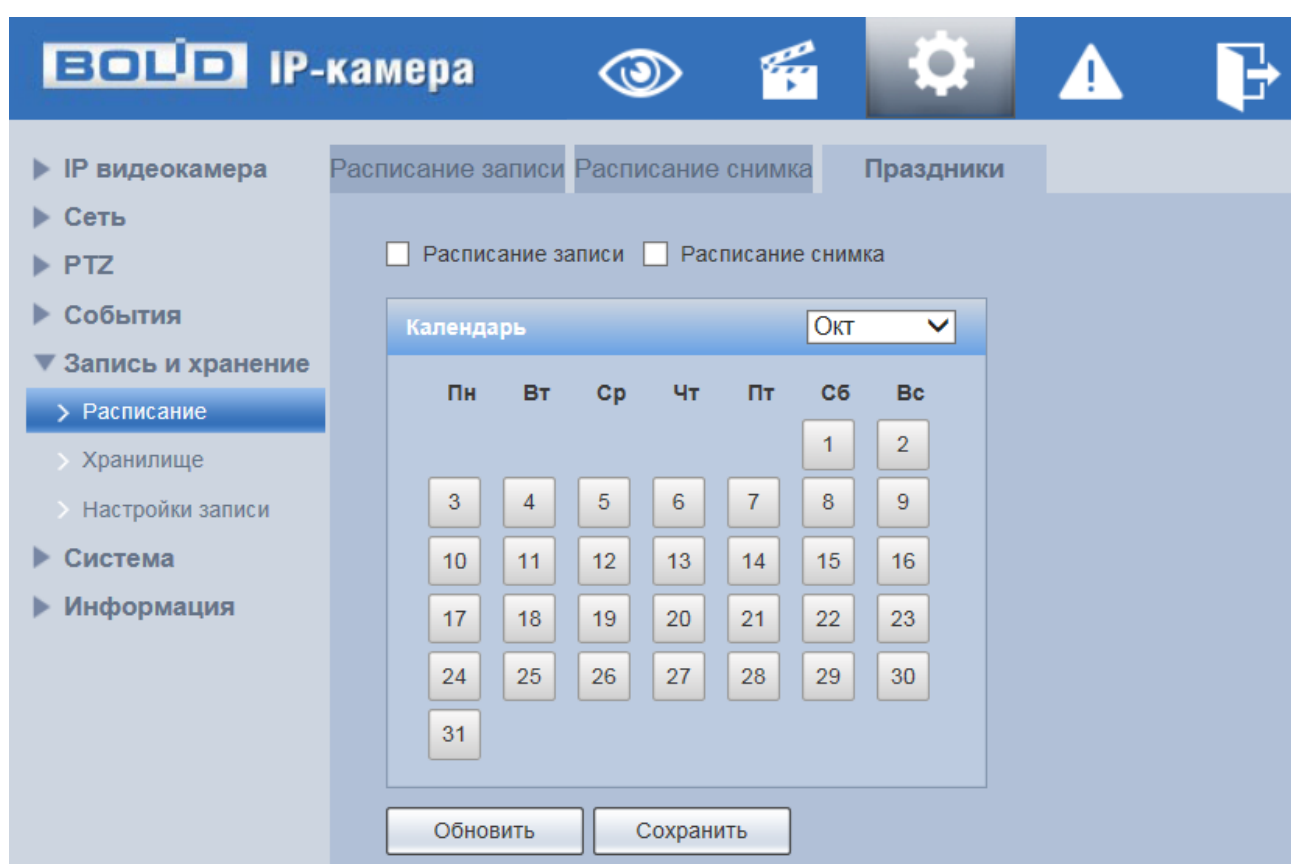
Рисунок 7.128 — Вкладка «Праздники»
