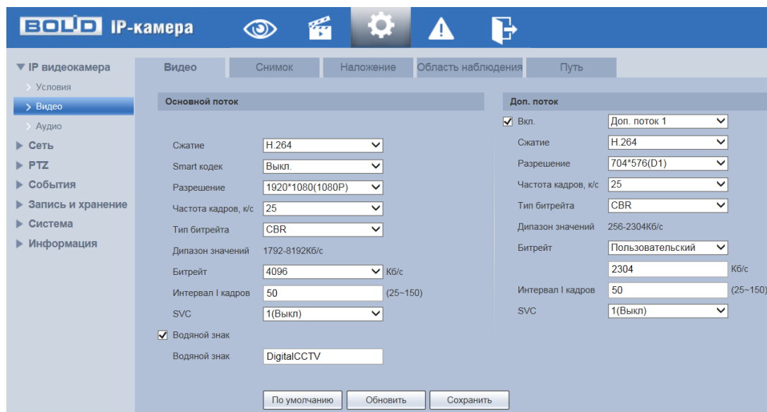
Рисунок 7.42 — Вкладка «Видео»
