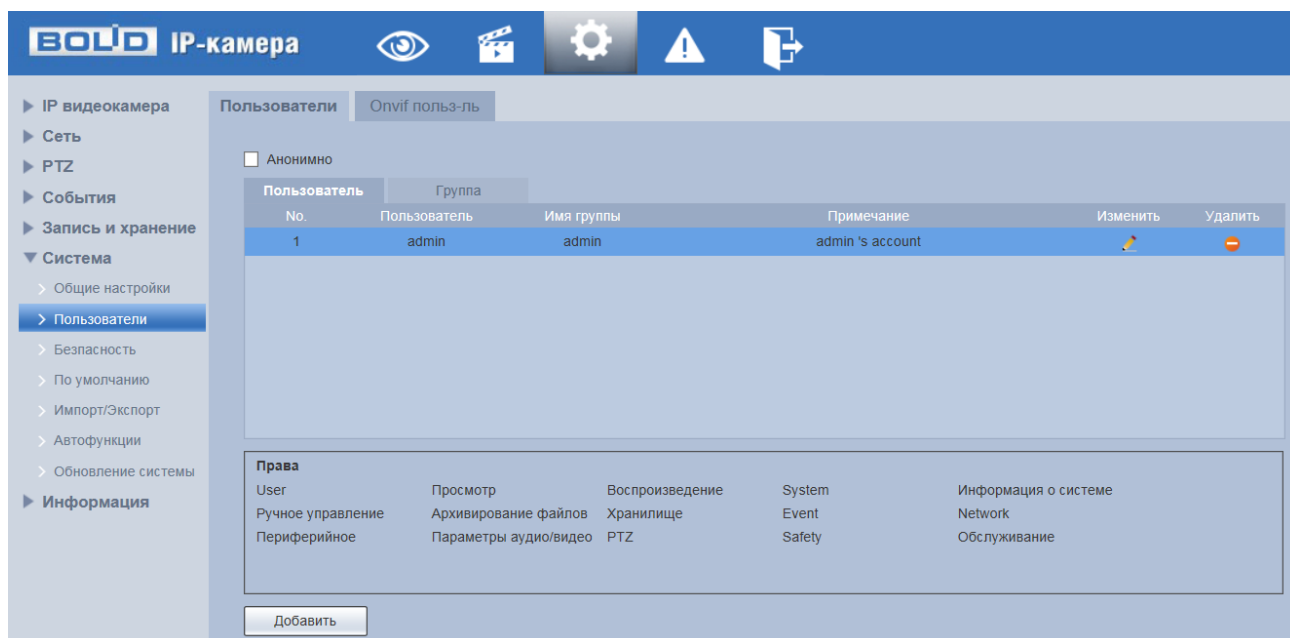
Рисунок 7.139 — Вкладка «Пользователи»
