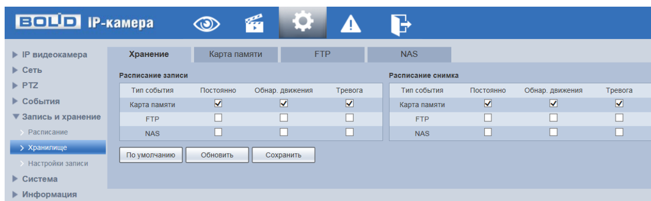
Рисунок 7.130 — Вкладка «Хранение»
