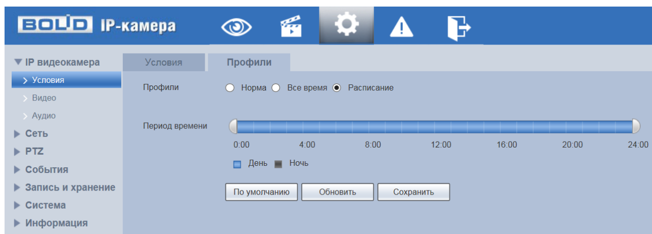
Рисунок 7.40 — Вкладка «Профили»
