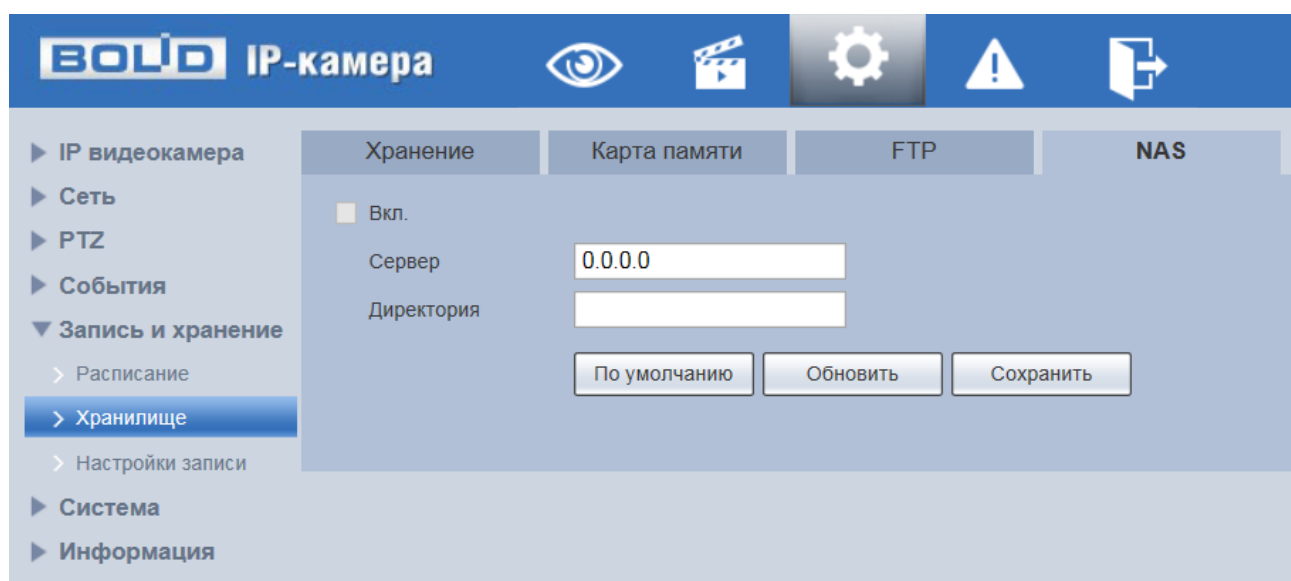
Рисунок 7.133 — Вкладка «NAS»
