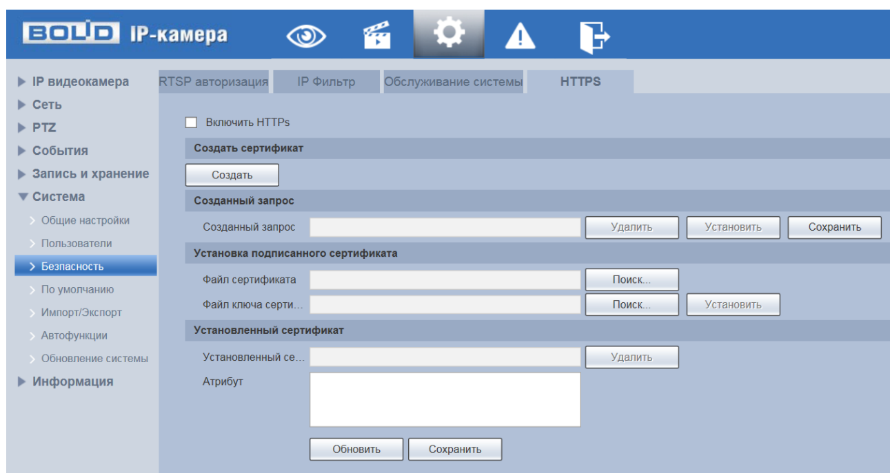
Рисунок 7.146 — Вкладка «HTTPS»
