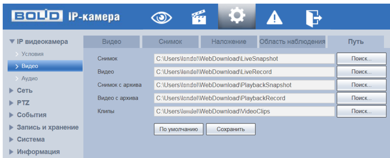
Рисунок 7.56 — Вкладка «Путь»
