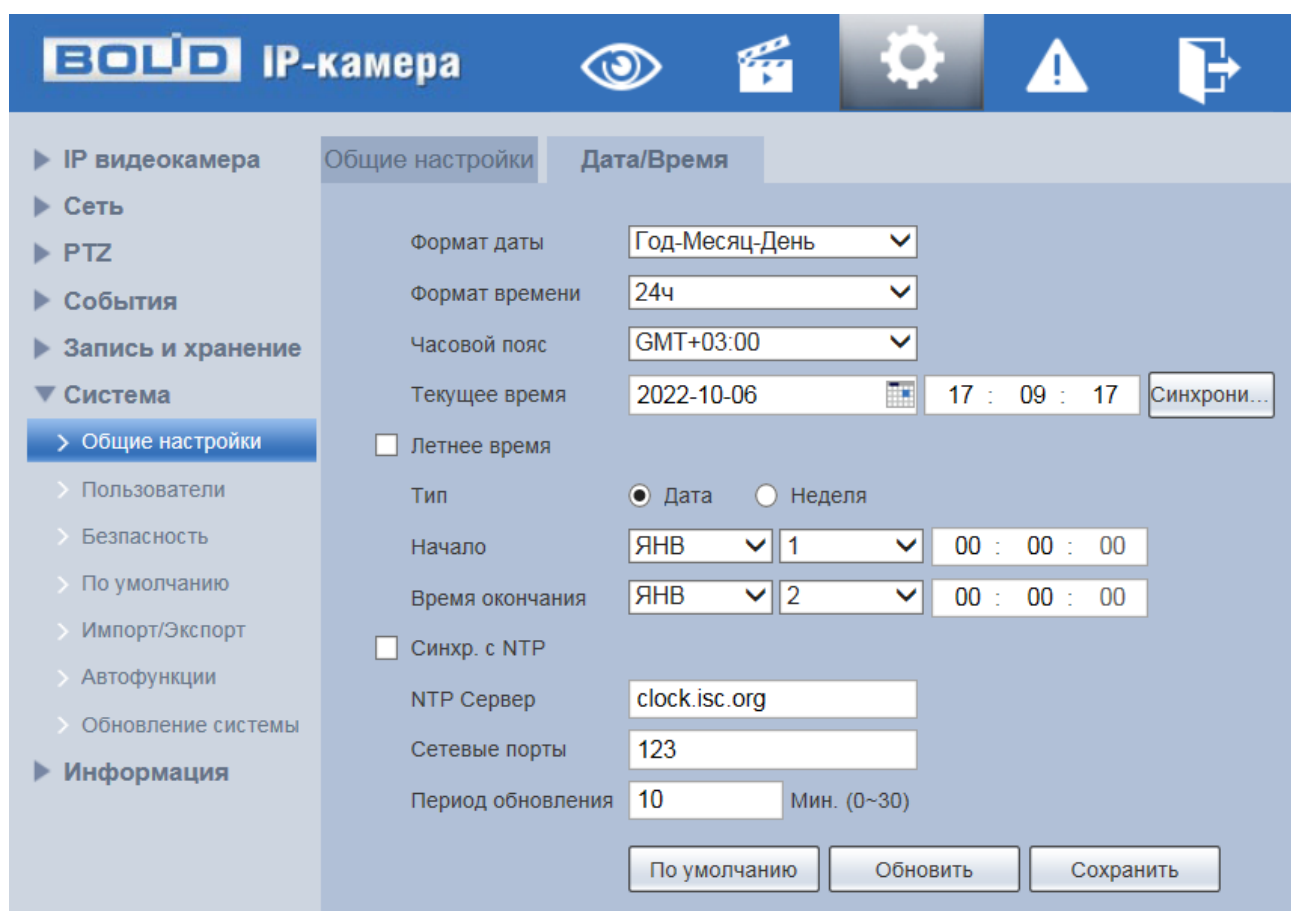
Рисунок 7.138 — Вкладка «Дата/Время»
