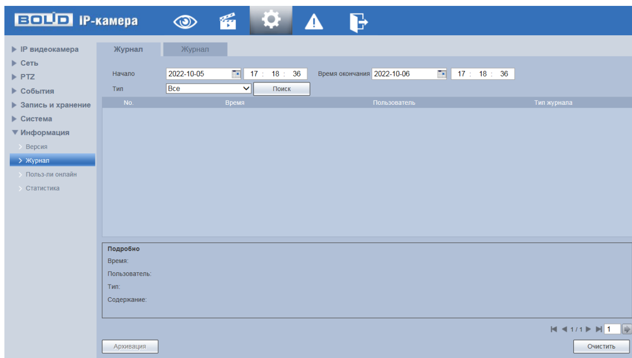
Рисунок 7.155 — Вкладка «Журнал»
