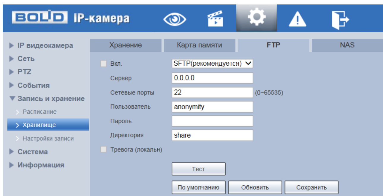
Рисунок 7.132 — Вкладка «FTP»
