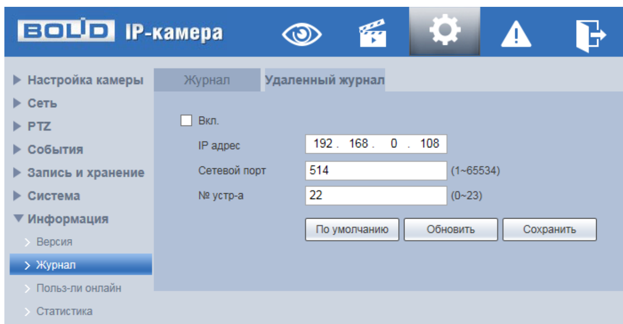
Рисунок 7.166 — Вкладка «Удаленный журнал»
