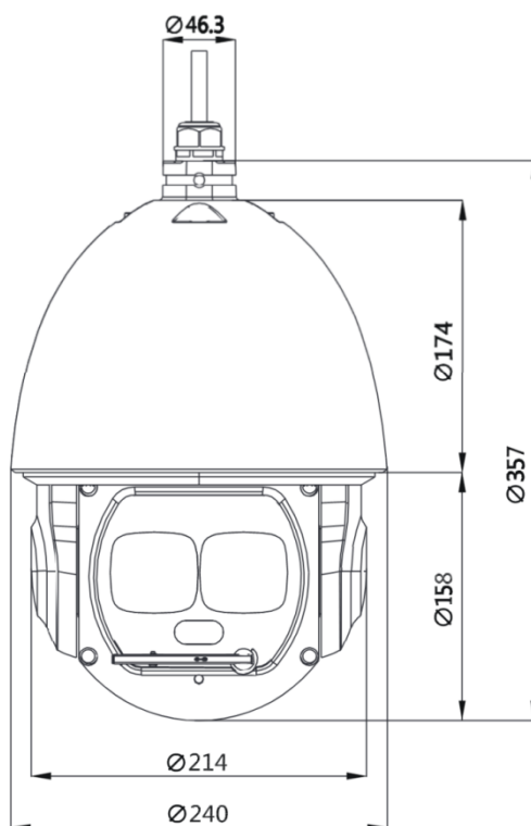
Рисунок 5.1 — Габаритные размеры видеокамеры (мм)
