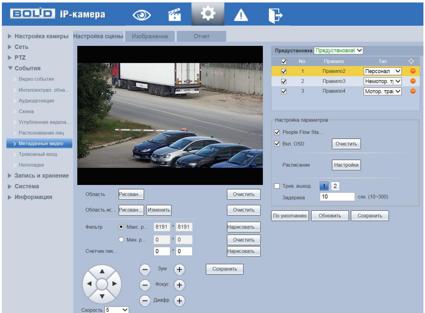
Рисунок 7.117 — Вкладка «Настройка сцены»
