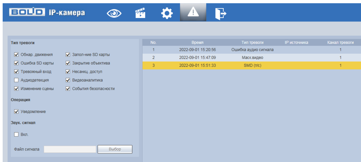
Рисунок 7.169 — Раздел меню «События»
