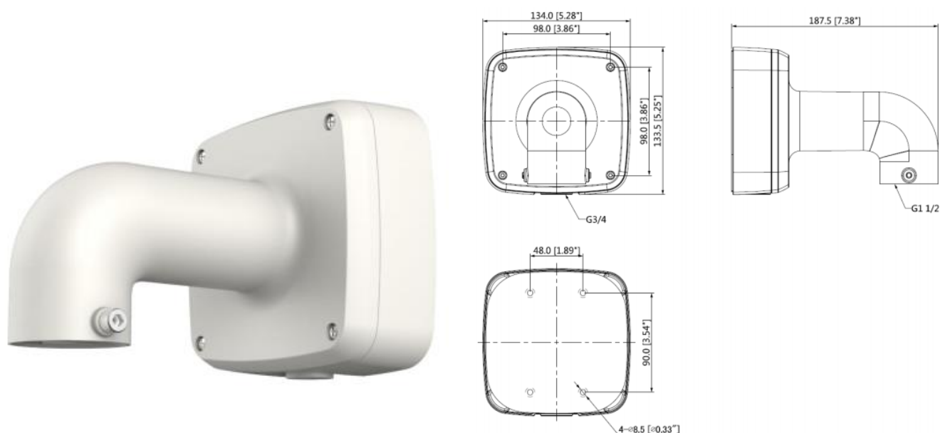
Рисунок 5.9 — Настенный кронштейн BR-107
