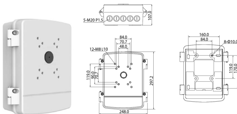
Рисунок 5.5 — Монтажная коробка BR-203
