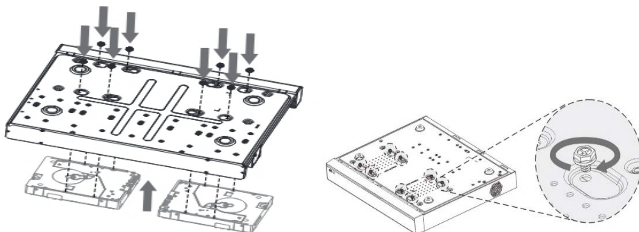
Рисунок 3.6 – Установка жесткого диска
