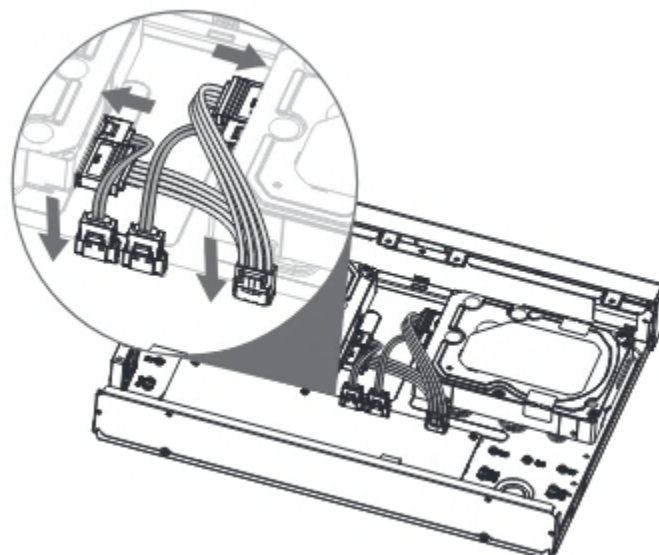
Рисунок 3.7 – Установка жесткого диска
