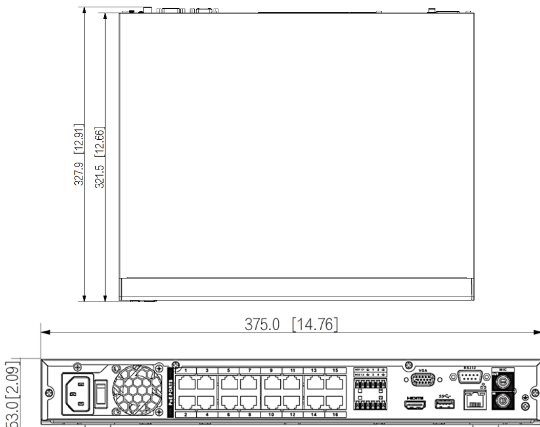
Рисунок 3.9 – Габаритные размеры видеорегистратора
