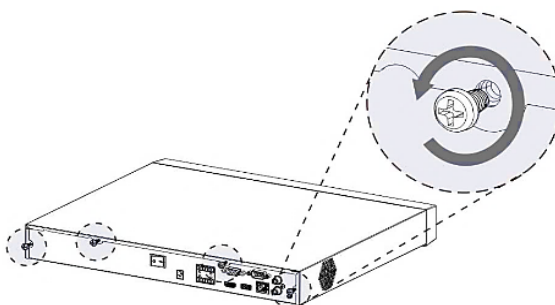
Рисунок 3.3 – Установка жесткого диска
