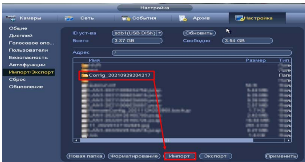
Рисунок 18.5 – Импорт настроек на видеорегистратор
