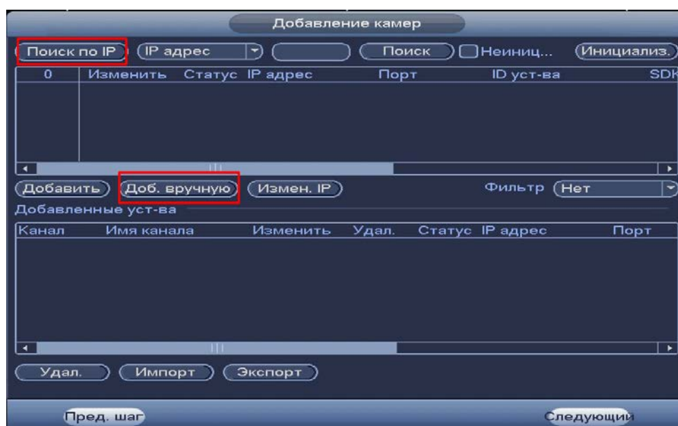
Рисунок 5.6 – Настройка добавления камер по поиску в сети
