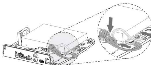
Рисунок 3.7 – Установка жесткого диска
