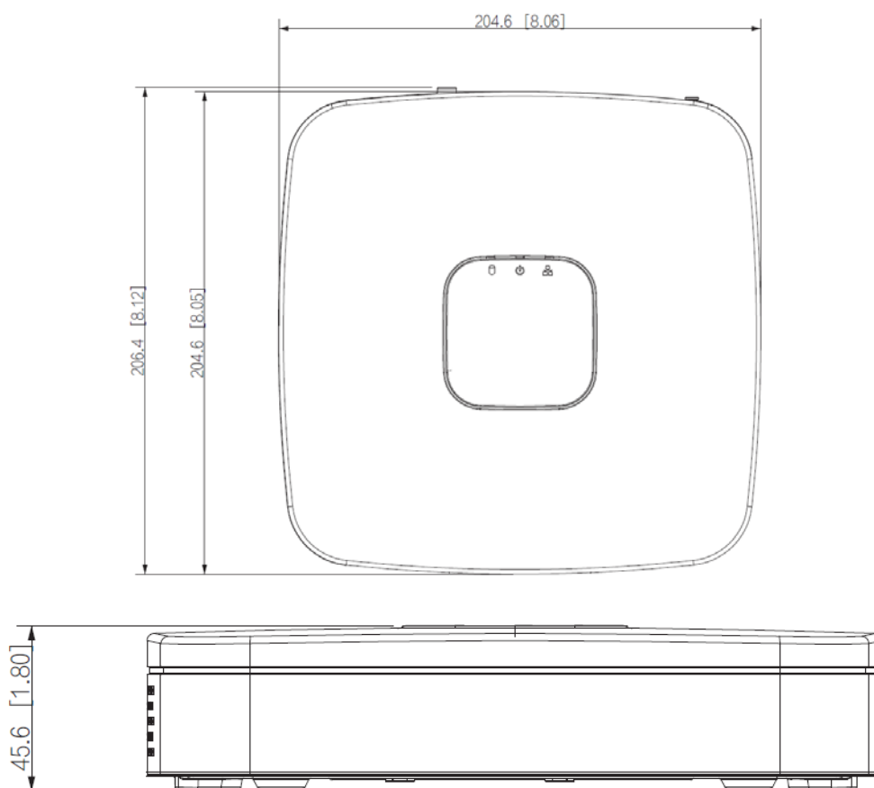
Рисунок 3.9 – Габаритные размеры видеорегистратора
