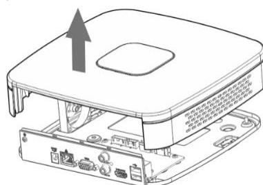
Рисунок 3.4 – Установка жесткого диска
