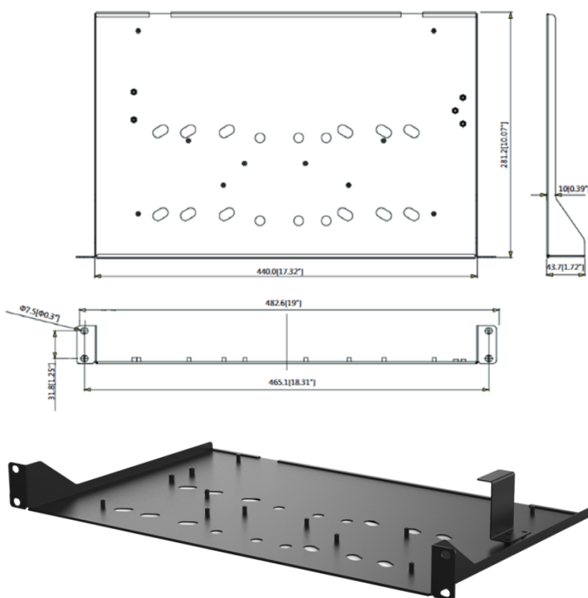
Рисунок 3.10 – Внешний вид и габариты BOLID BR-111
