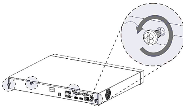
Рисунок 3.3 – Установка жесткого диска
