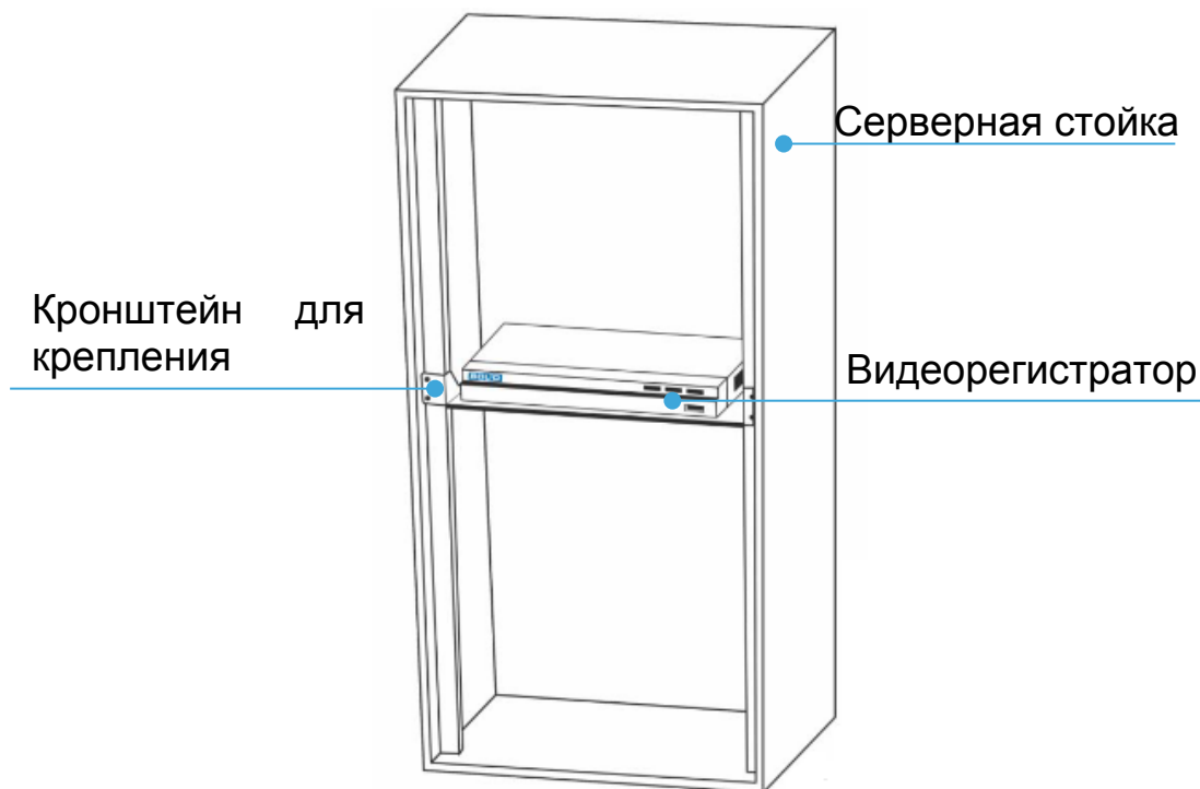
Рисунок 3.11 – Монтаж видеорегистратора в 19” - стойку с помощью кронштейна
