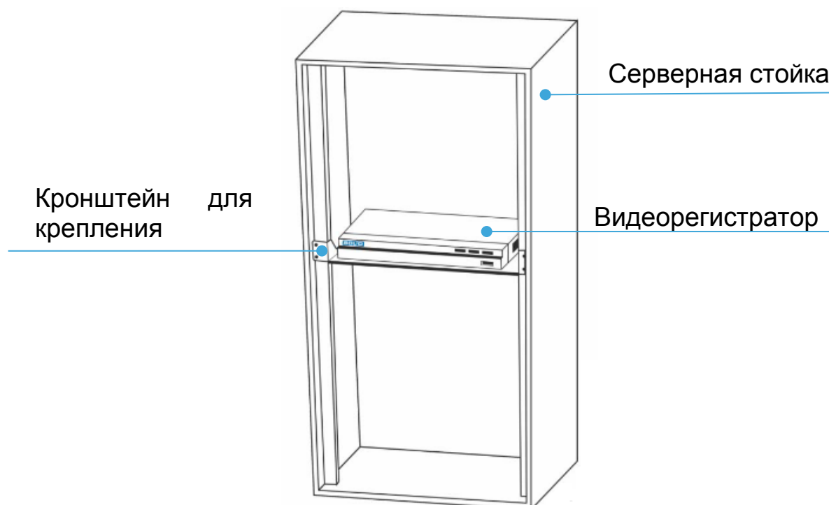
Рисунок 3.11 – Монтаж видеорегистратора в 19” - стойку с помощью кронштейна
