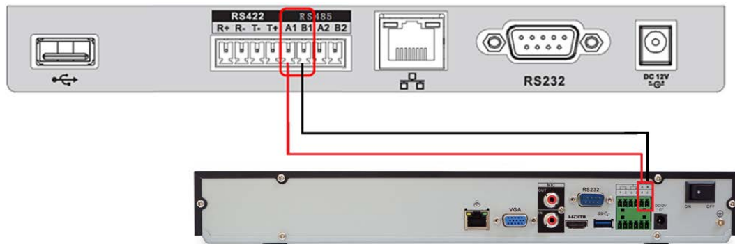
Рисунок 12.4 – Схема RS-485
