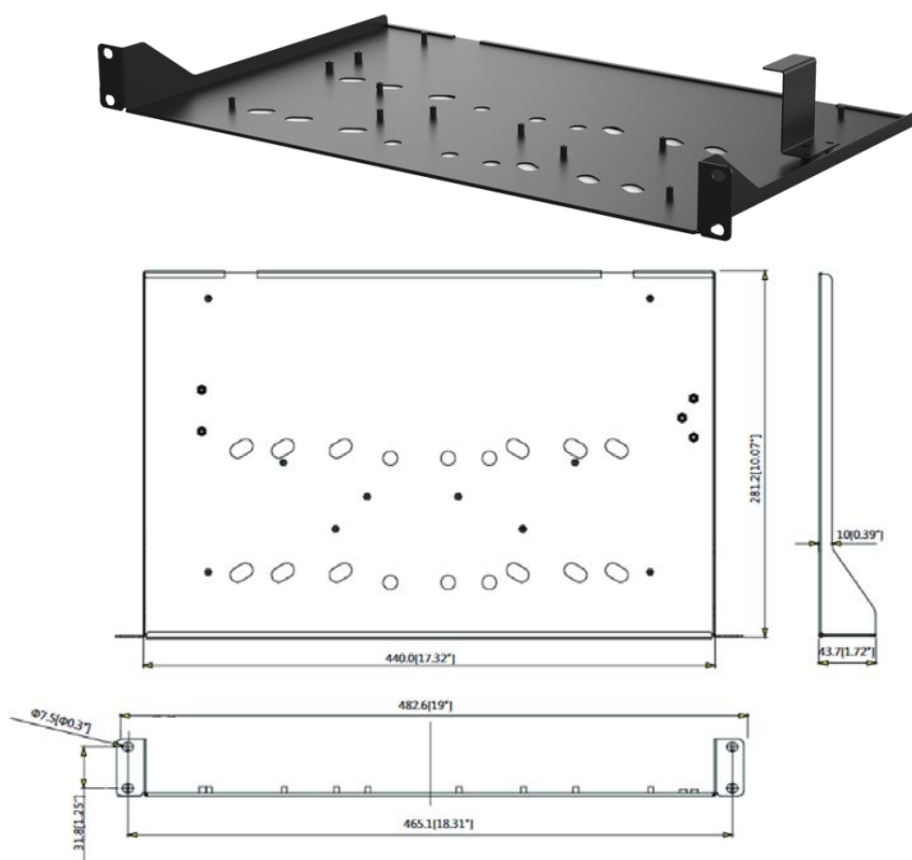
Рисунок 3.10 – Внешний вид и габариты BOLID BR-111 Основные характеристики кронштейна для крепления BOLID BR-111
