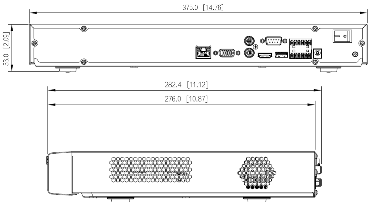
Рисунок 3.9 – Габаритные размеры видеорегистратора
