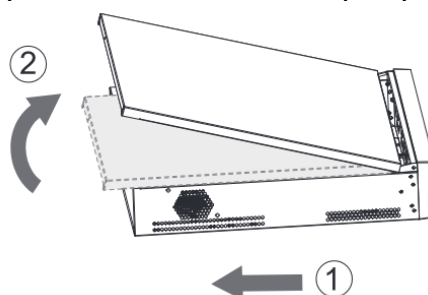
Рисунок 3.4 – Установка жесткого диска
