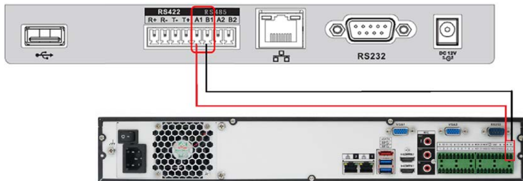
Рисунок 12.4 – Схема RS-485
