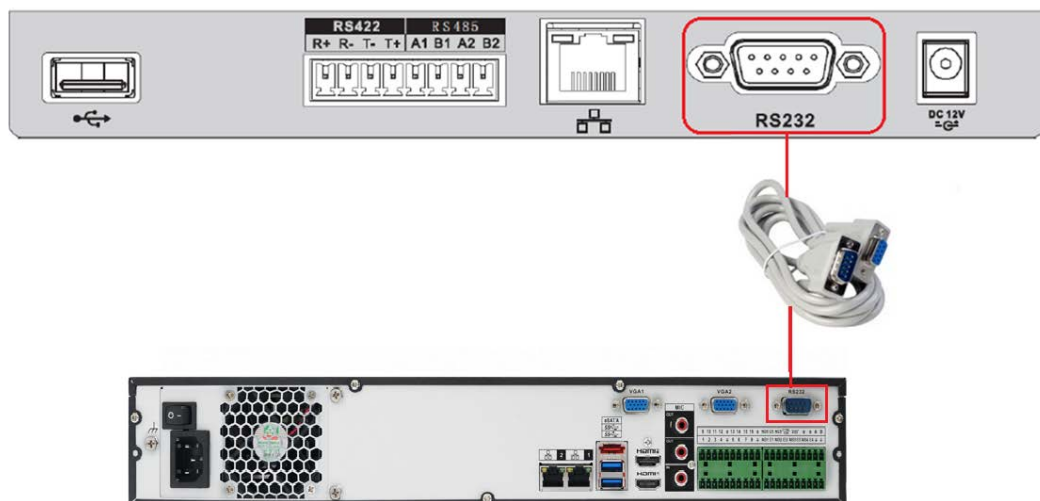
Рисунок 12.5 – Схема RS-232
