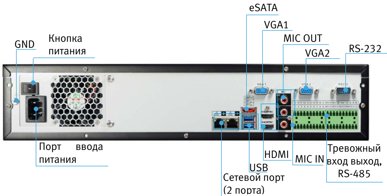
Рисунок 3.2 – Внешний вид задней панели корпуса
