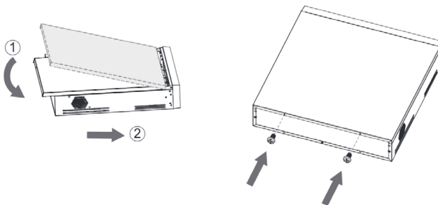
Рисунок 3.9 – Установка жесткого диска
