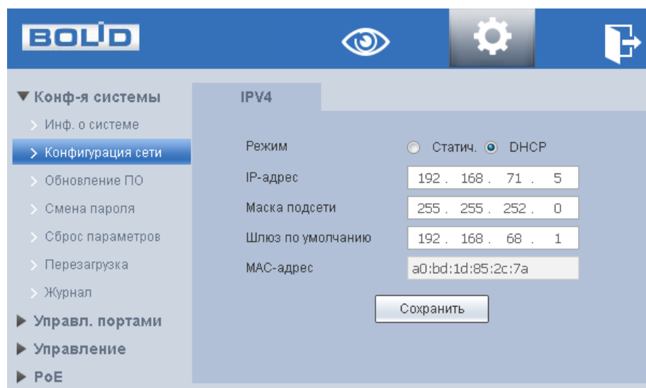
Рисунок 6.4 – Сетевые настройки
