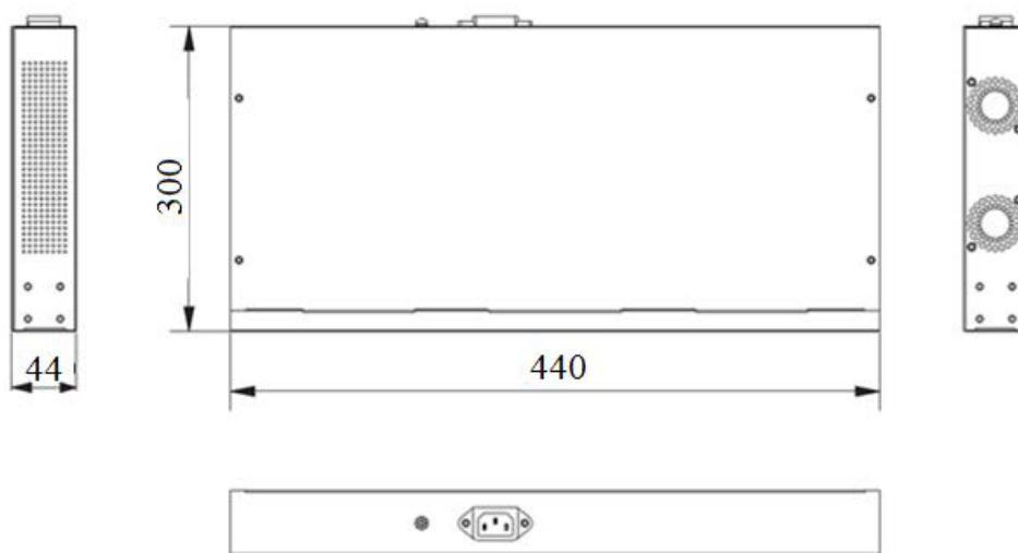
Рисунок 4.4 – Габаритные размеры
