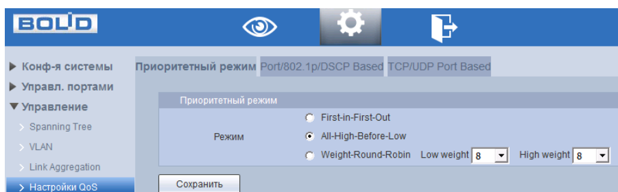
Рисунок 6.24 – Приоритетный режим
