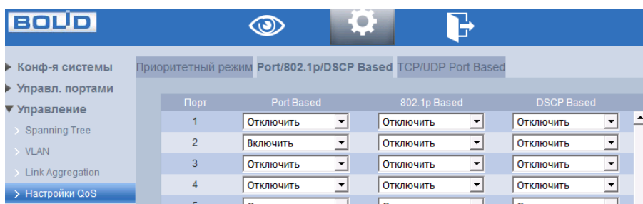
Рисунок 6.25 – Приоритетный режим
