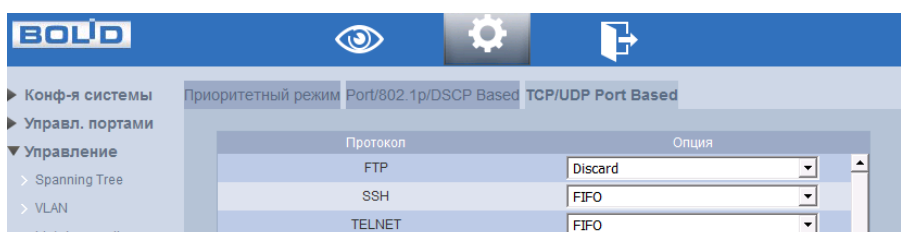
Рисунок 6.26 – Задайте «Discard»
