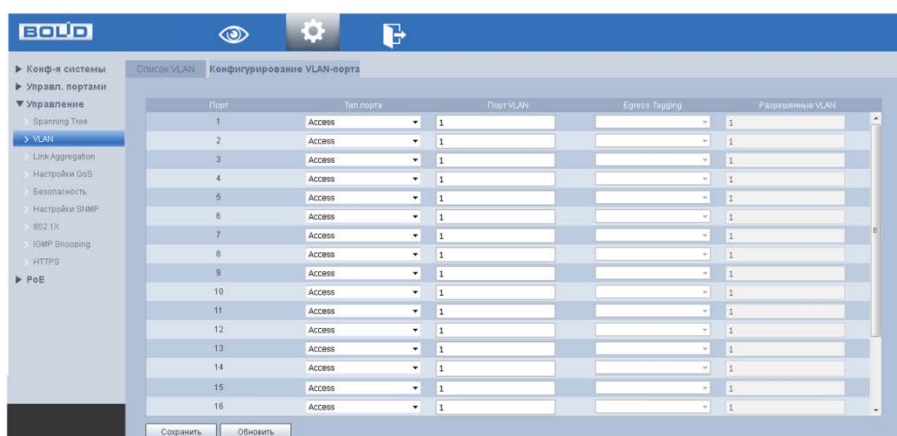
Рисунок 6.20 – Конфигурирование VLAN-порта
