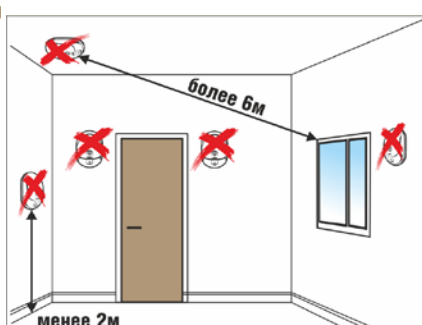
Рисунок 2.2.3.2.6 НЕрекомендуемые места установки извещателя
