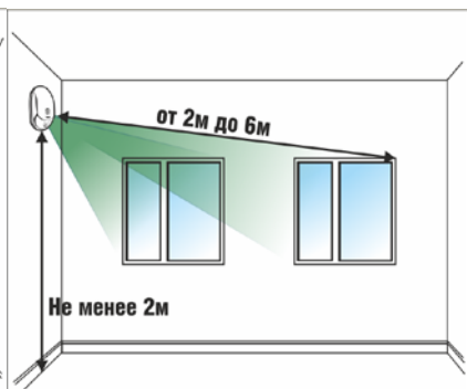
Рисунок 2.2.3.2.2 Установка извещателя на боковой стене
