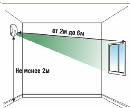
Рисунок 2.2.3.2.3 Установка извещателя на противоположной стене
