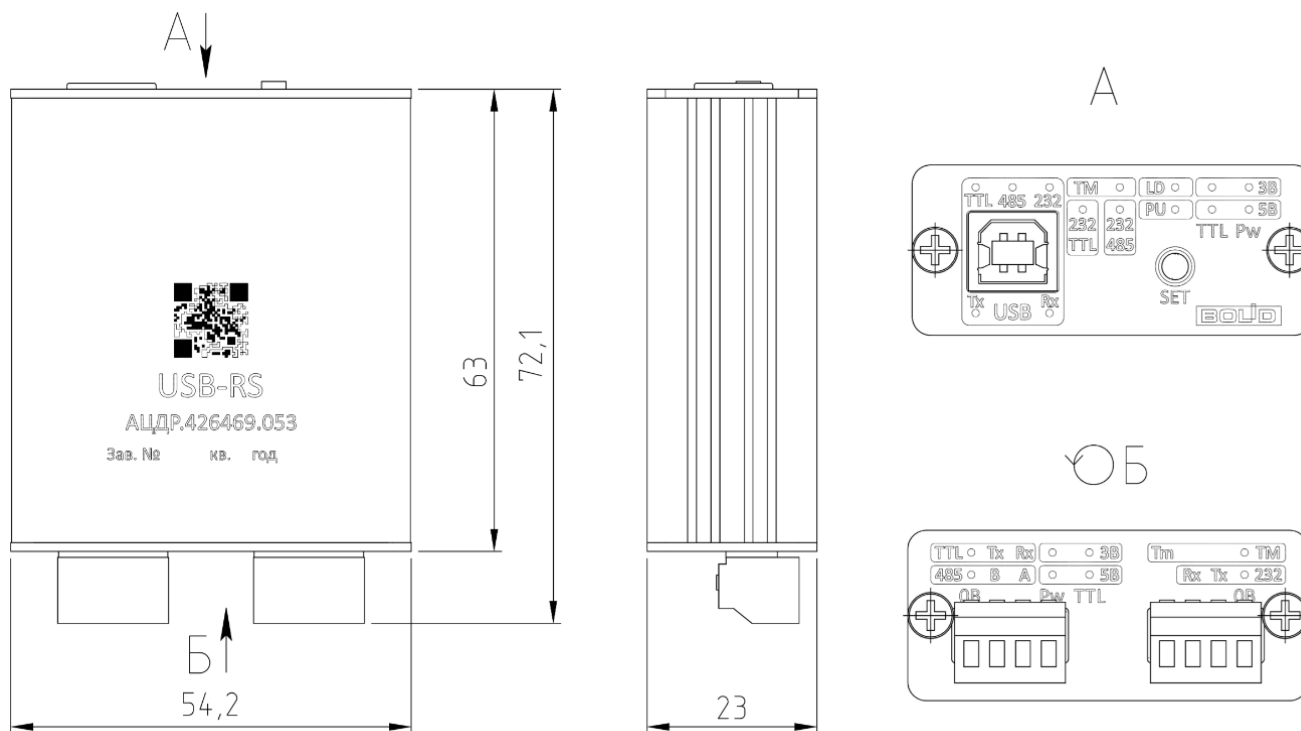
Рис.2.1 Внешний вид и габаритные размеры преобразователя «USB-RS»
