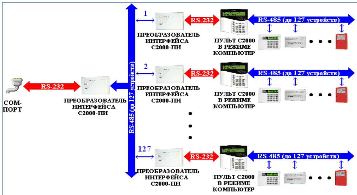
Схема подключения нескольких веток приборов к одному COM-порту/USB-порту компьютера по протоколу «Орион Про».
