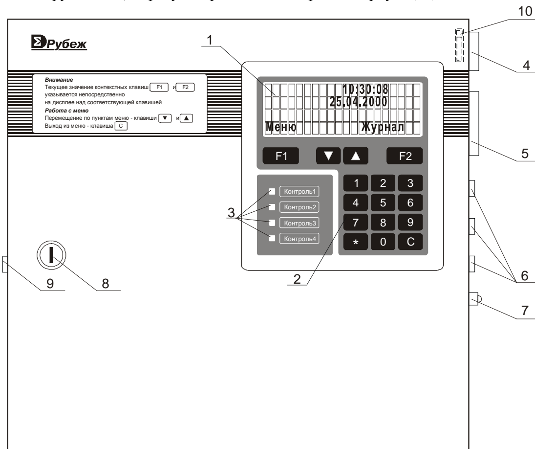
Рис. 8 Внешний вид БЦП исп.3
