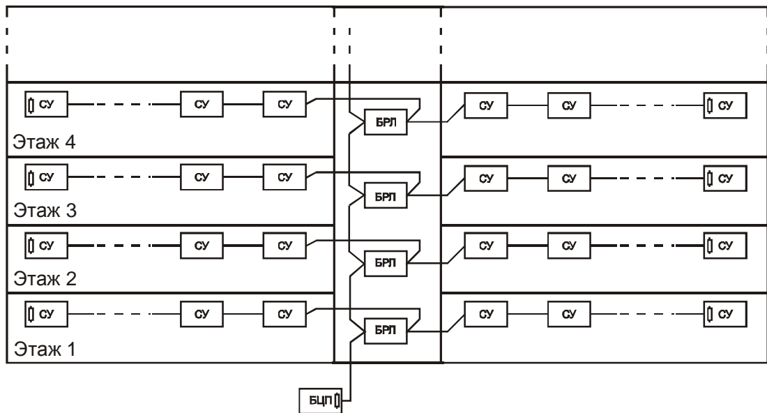
Рис. 16 Типовой вариант включения СУ
