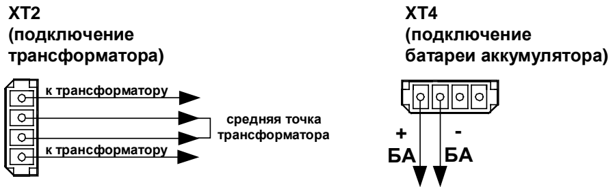
Рис. 30 Разъемы XT2 и XT4 исп. 3
