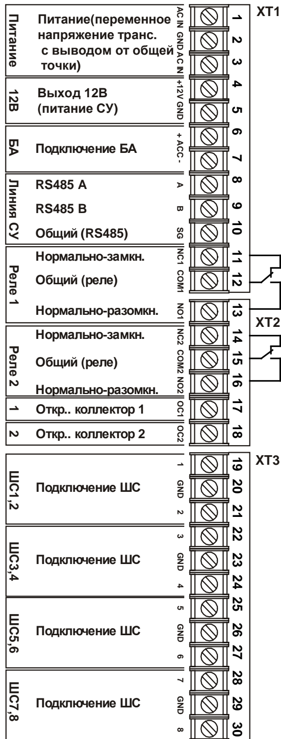
Рис. 35 Назначение разъемов ХТ1, ХТ2, ХТ3 БЦП исп.4
