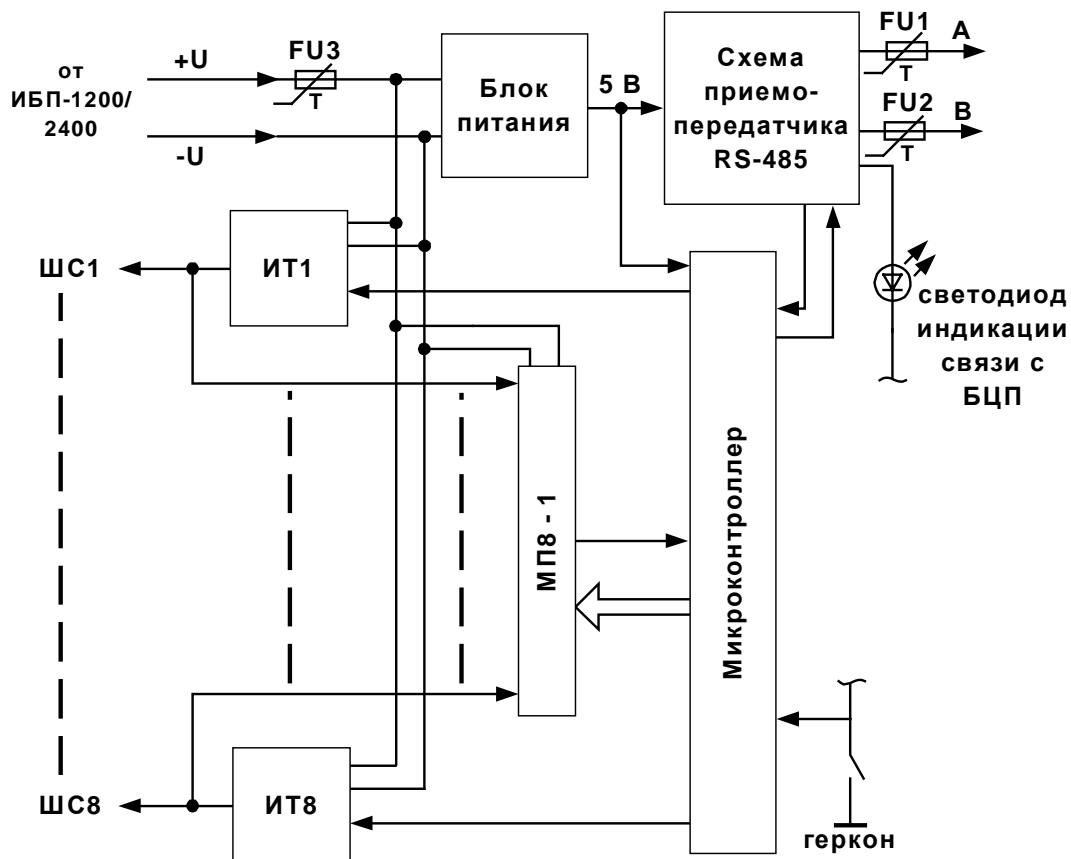
Рис. 2 Схема электрическая структурная СКШС
