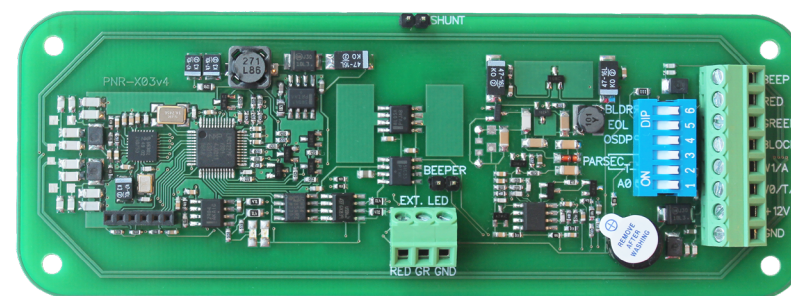
Рисунок 1. Считыватель PNR-X03E
