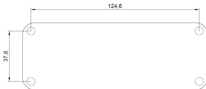
PNR-X03E
