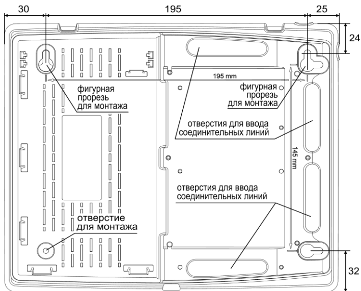
Рис.3 Задняя стенка прибора. Присоединительные размеры
