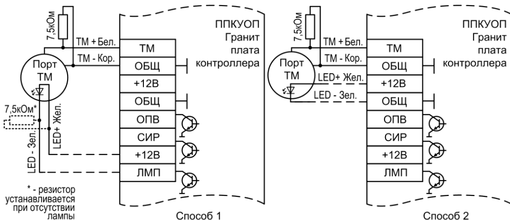
Рис.Б1 Схемы подключения порта ТМ
