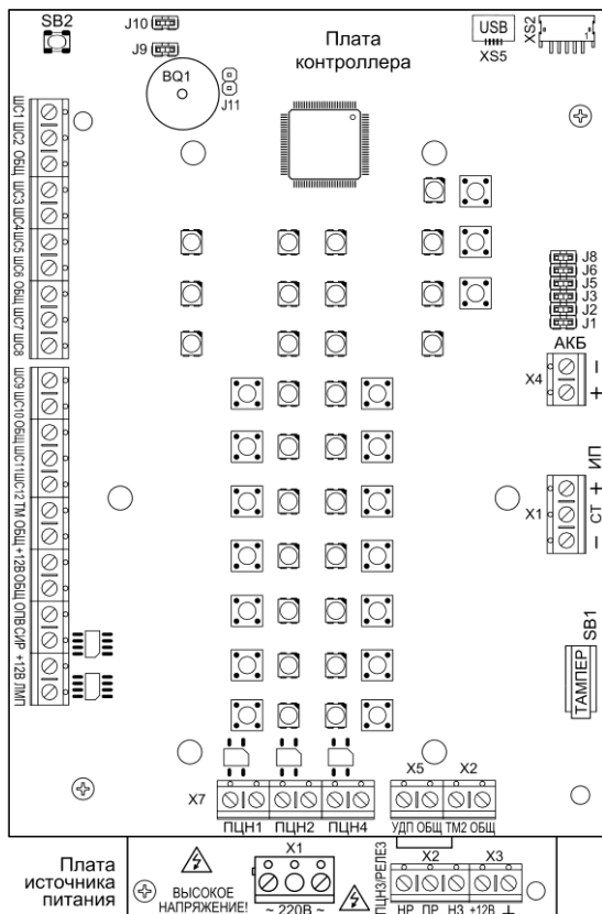
Рис.1 Плата контроллера Гранит-12 (вид со снятой панелью индикации и управления) и плата источника питания (видимая часть)
