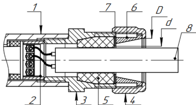
Рис.3 Конструкция и обеспечение взрывозащиты датчика Ех ДВГ 102
