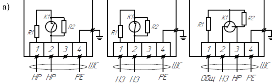
Рис.5 Электрическая схема датчиков Ex ДВГ 102
