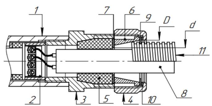
Рис.3 Конструкция и обеспечение взрывозащиты датчика Ех ДВГ 102
