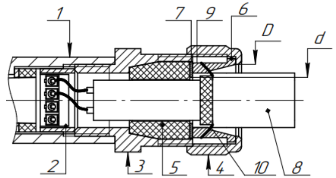
Рис.4.4 установка бронекабеля диам. подключаемого кабеля 6-18мм 1.Корпус датчика; 2.Клеммная колодка; 3.Корпус ввода; 4.Гайка; 5.Уплотнитель; 6.Втулка; 7.Шайба; 8.Кабель, 9. Конус, 10.броня
