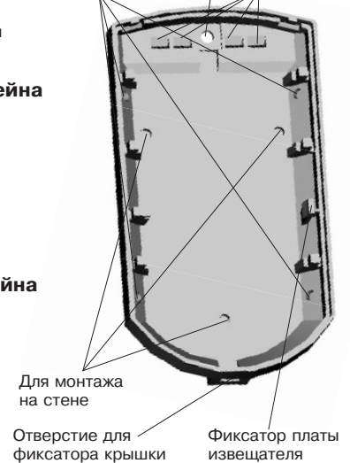
Рисунок 2 – Основание извещателя и кронштейн
