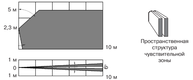
Рисунок 1 – Диаграмма зоны обнаружения
