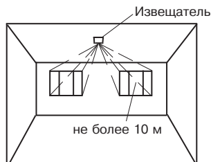
Рисунок 3 – Установка извещателя на потолок
