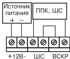
Рисунок 3 – Схема подключения извещателя с объединенными шлейфами сигнализации и вскрытия корпуса
