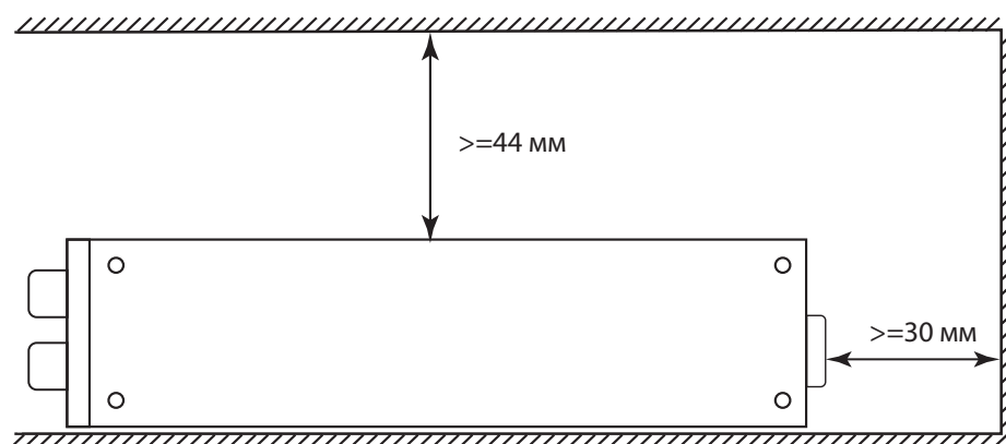
Рис.3. Установка усилителя
