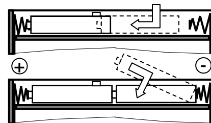
Установка первой пары элементов питания
